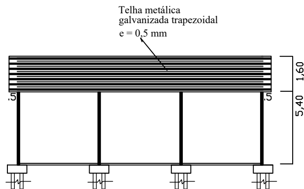
Corte BB Esc.: 1/100
