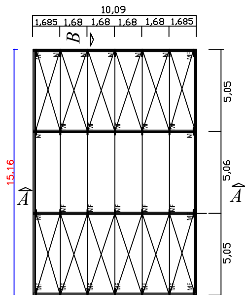
PLANTA DE FÔRMA DA ESTRUTURA Esc.: 1/100
