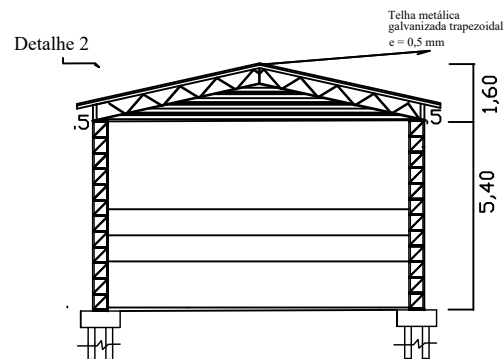
Corte AA Esc.: 1/100
