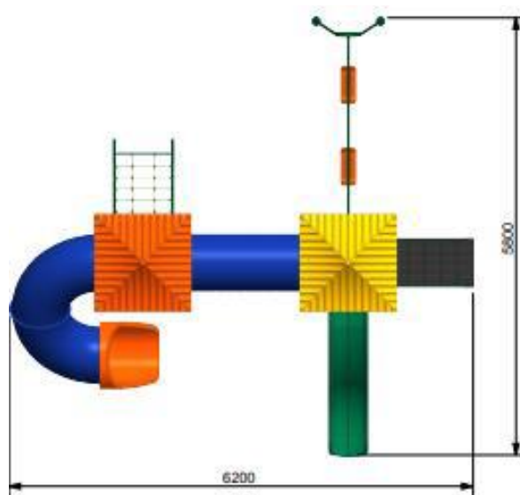
Figura 4 - Vista em planta
