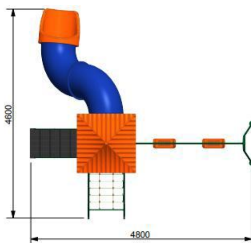
Figura 2 - Vista em planta
