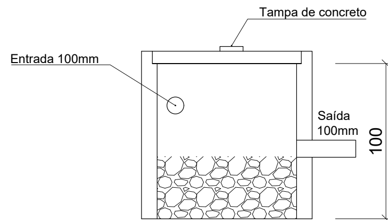
3 CORTE F-F ESCALA 1:25
