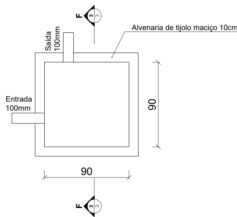
2 PLANTA CAIXA PASSAGEM ESCALA 1:25
