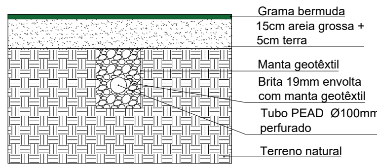
4 DETALHE DRENAGEM ESCALA 1:25
