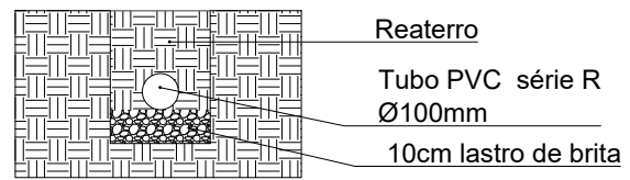
5 DETALHE DRENAGEM TUBO PVC CÓRREGO ESCALA 1:25
