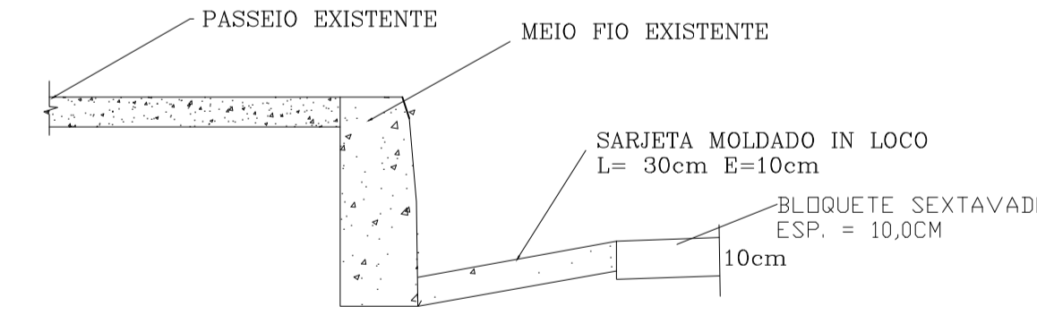
DETALHE CONSTRUTIVO DO MEIO FIO E SARJETA SEM ESCALA
