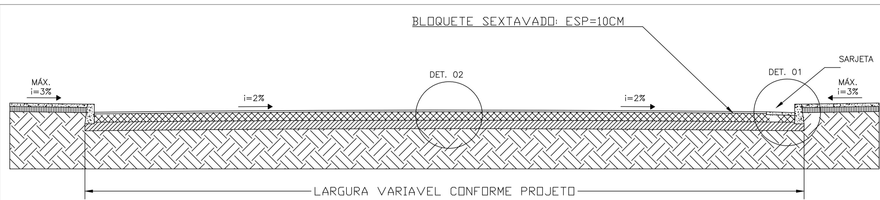
SEÇÃO BÁSICA DAS VIAS ESCALA 1:50
