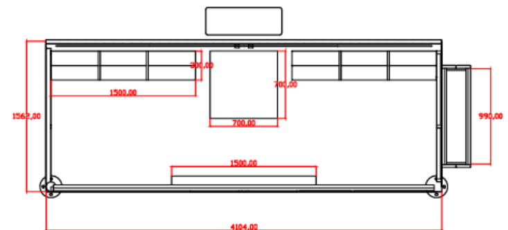
PLANTA BAIXA
