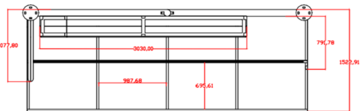
PLANTA BAIXA
