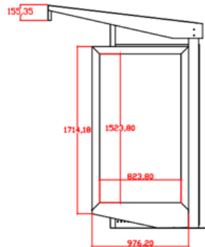
VISTA DIREITA
