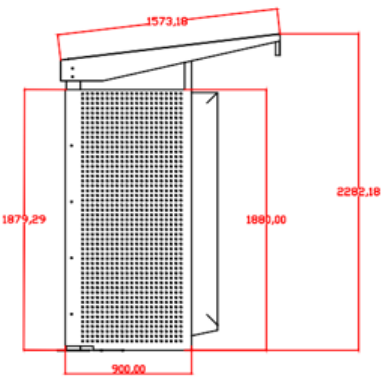
VISTA ESQUERDA
