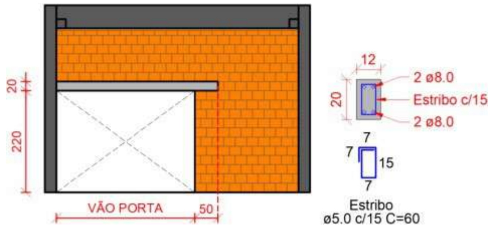
Figura 04 – Exemplo vergas
