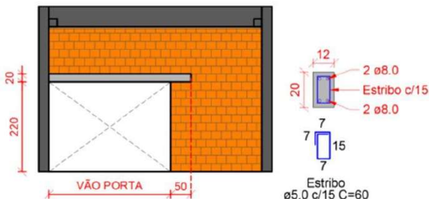
Figura 03: Exemplo vergas.
