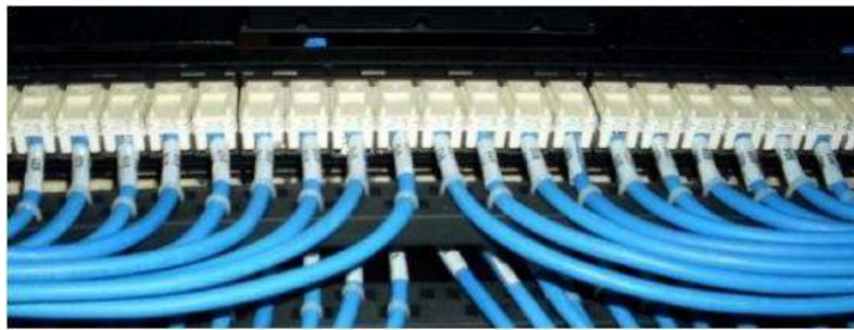
Figura 06 - Fixação do cabeamento permanente no painel de conexão.
