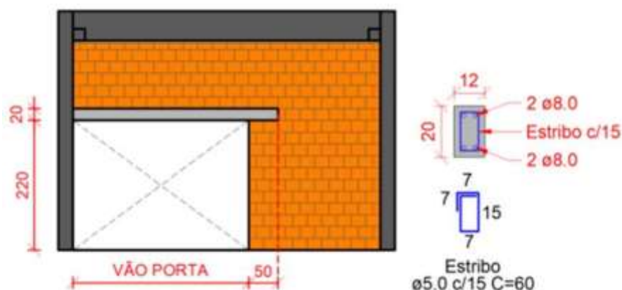
Figura 03: Exemplo vergas.
