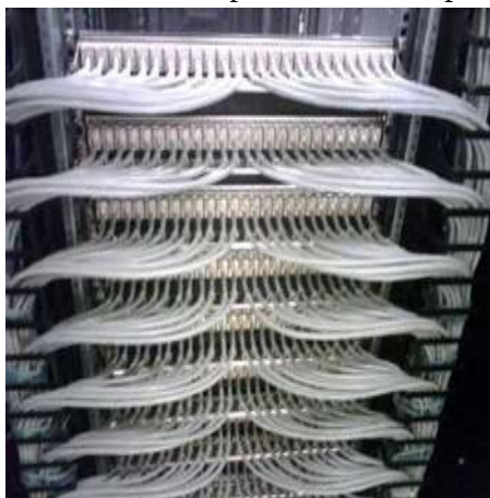
Figura 05 - Fixação do cabeamento permanente no painel de conexão.
