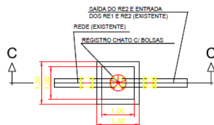
DETALHE 3 TÍPICO
