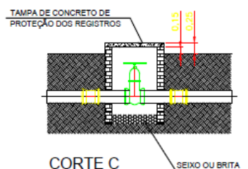
CORTE C
