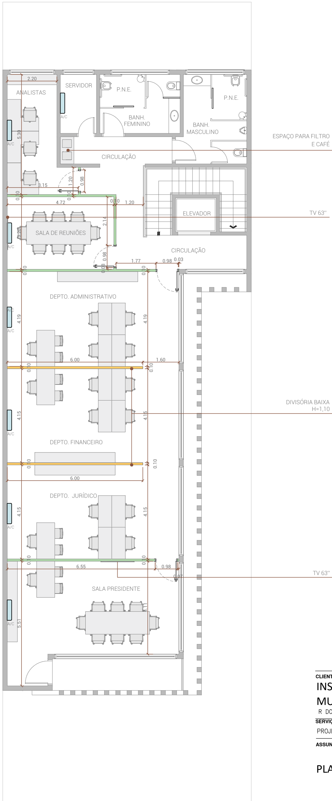
PLANTA SUPERIOR ESC. 1:100
