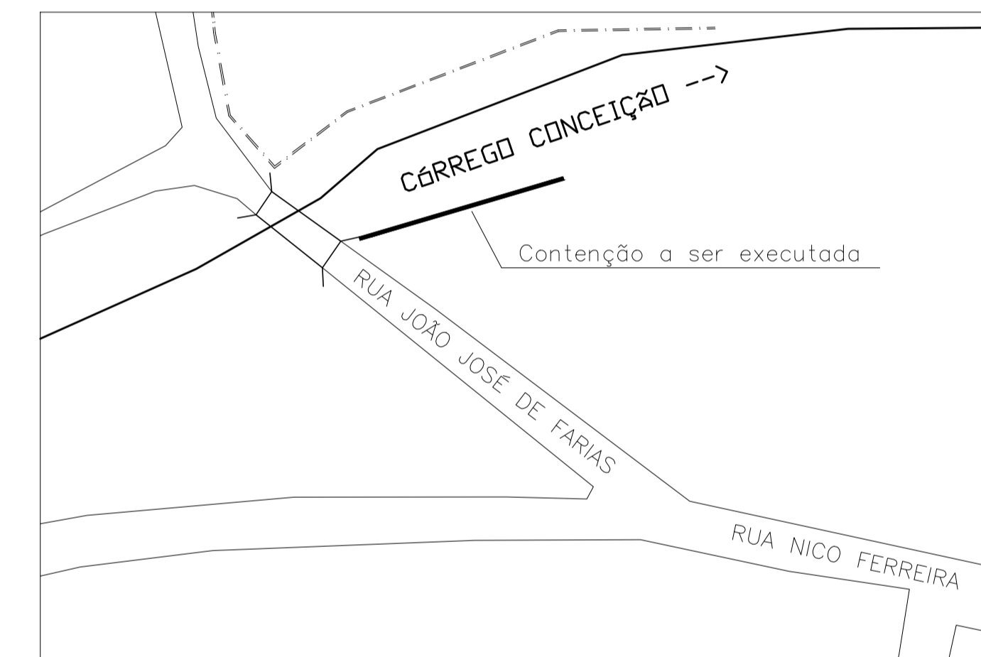
PLANTA DE LOCAÇÃO sem escala
