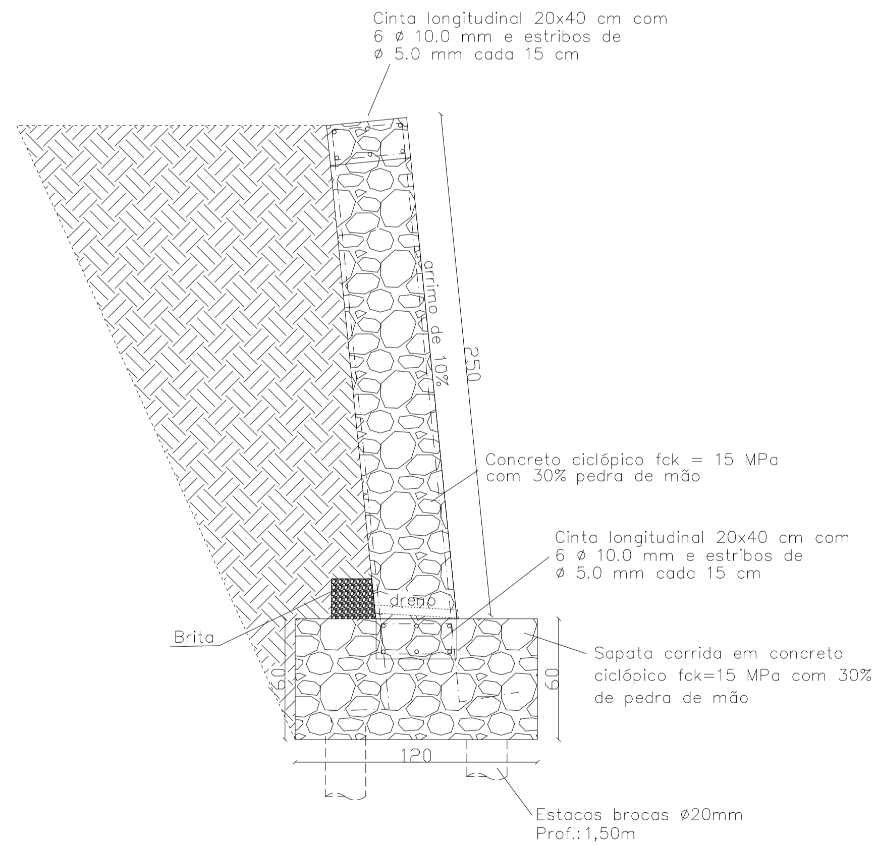
MURO DE CONTENÇÃO SEÇÃO TÍPICA - FORMA E ARMAÇÃO ESCALA 1:50
