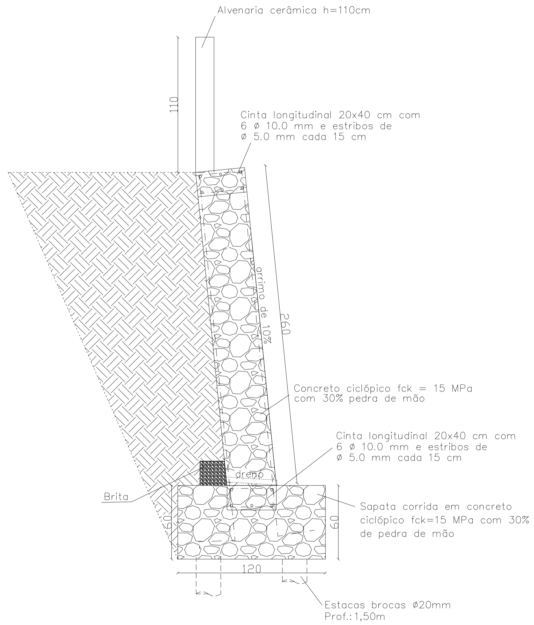
MURO DE CONTENÇÃO SEÇÃO TÍPICA - FORMA E ARMAÇÃO ESCALA 1:50
