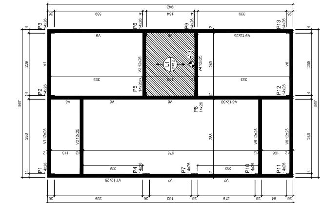
Forma do pavimento Nivel 1 Teto (Nivel 265) escala 1:50
