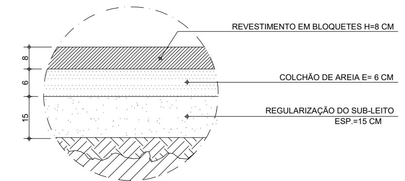
DETALHE 1- CORTE CAMADAS - BLOQUETE sem escala
