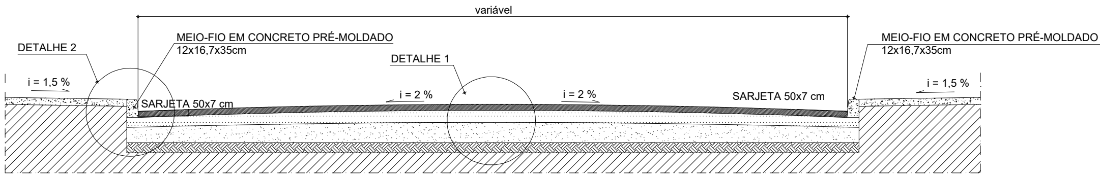
CORTE TRANSVERSAL – PISTA DE ROLAMENTO – BLOQUETE sem escala
