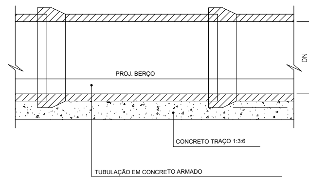
DETALHE INTERLIÇÃO TUBOS sem escala
