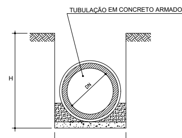
CORTE TRANSVERSAL DE VALAS sem escala
