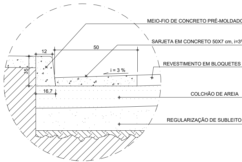
DETALHE 2- MEIO FIO E SARJETA- BLOQUETE sem escala
