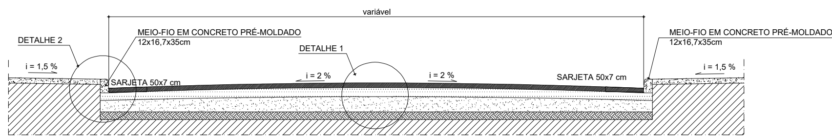
CORTE TRANSVERSAL - PISTA DE ROLAMENTO - BLOQUETE sem escala
