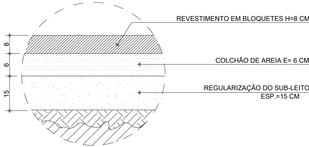
DETALHE 1- CORTE CAMADAS – BLOQUETE sem escala
