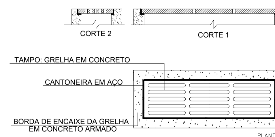
DETALHE DA GRELHA sem escala
