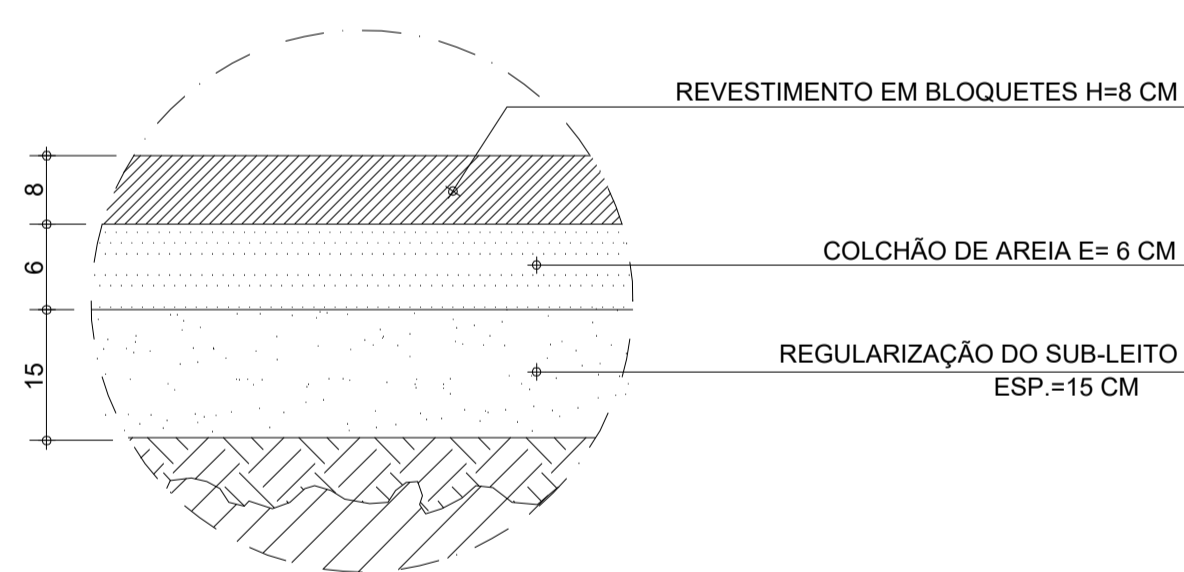
DETALHE 1- CORTE CAMADAS - BLOQUETE sem escala
