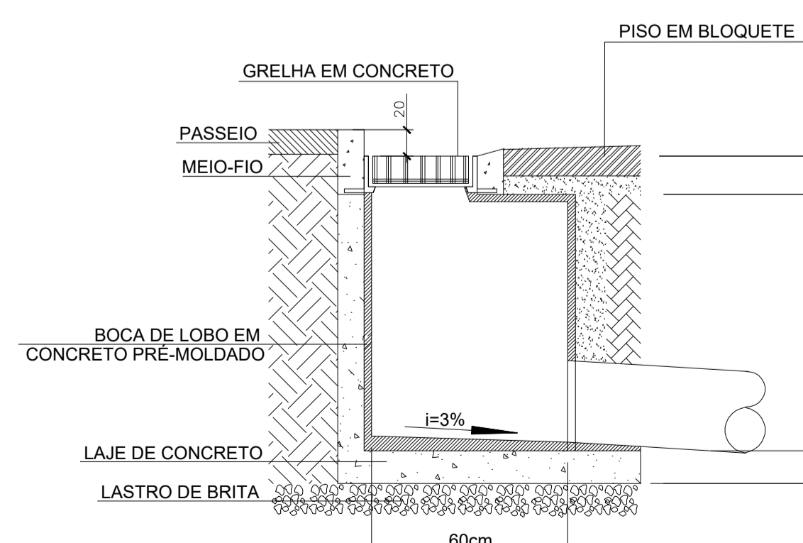
DETALHE BOCA DE LOBO sem escala
