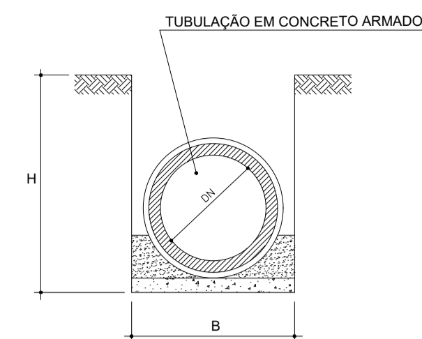
CORTE TRANSVERSAL DE VALAS sem escala
