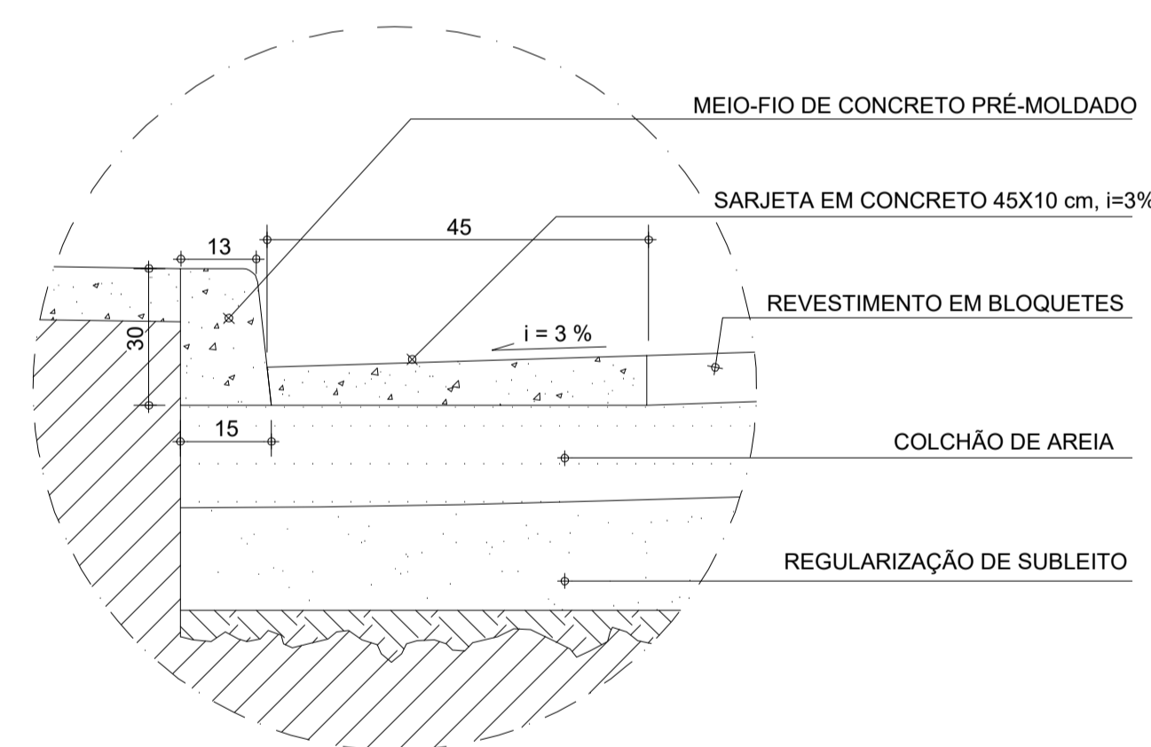
DETALHE 2- MEIO FIO E SARJETA- BLOQUETE sem escala
