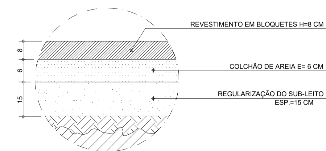
DETALHE 1- CORTE CAMADAS – BLOQUETE sem escala
