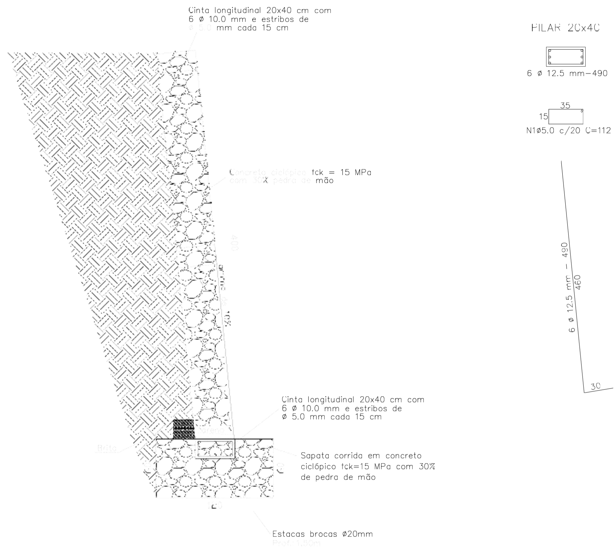
MURO DE CONTENÇÃO SEÇÃO TÍPICA - FORMA E ARMAÇÃO ESCALA 1:50
