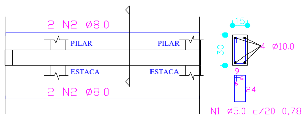
DETALHE VERGA E CONTRAVERGA
