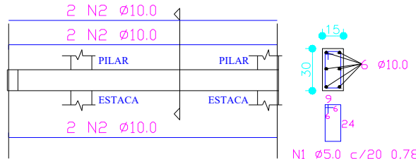
DETALHE VIGA COBERTURA
