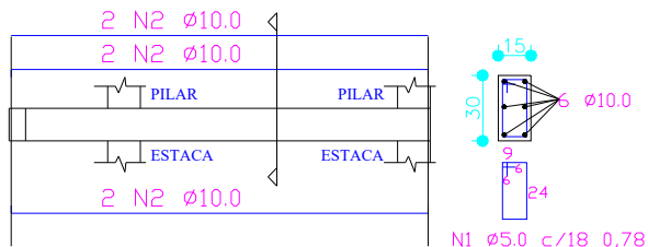
DETALHE VIGA BALDRAME
