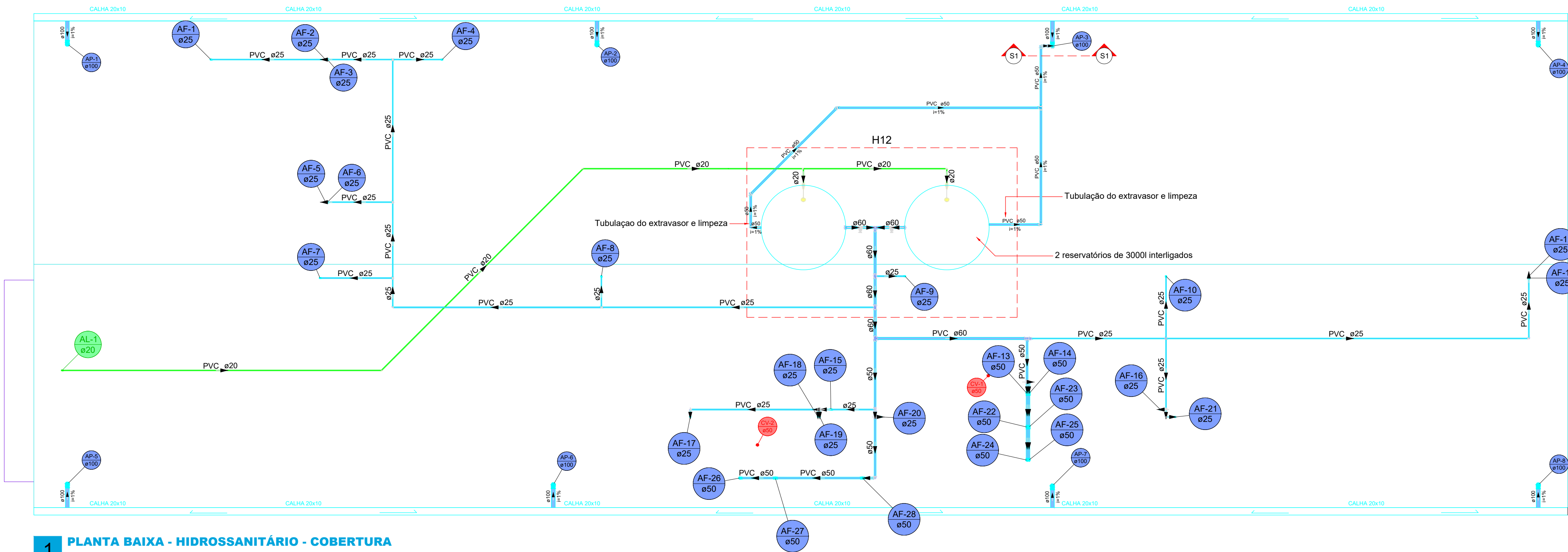
1 PLANTA BAIXA - HIDROSSANITÁRIO - COBERTURA 1:75
