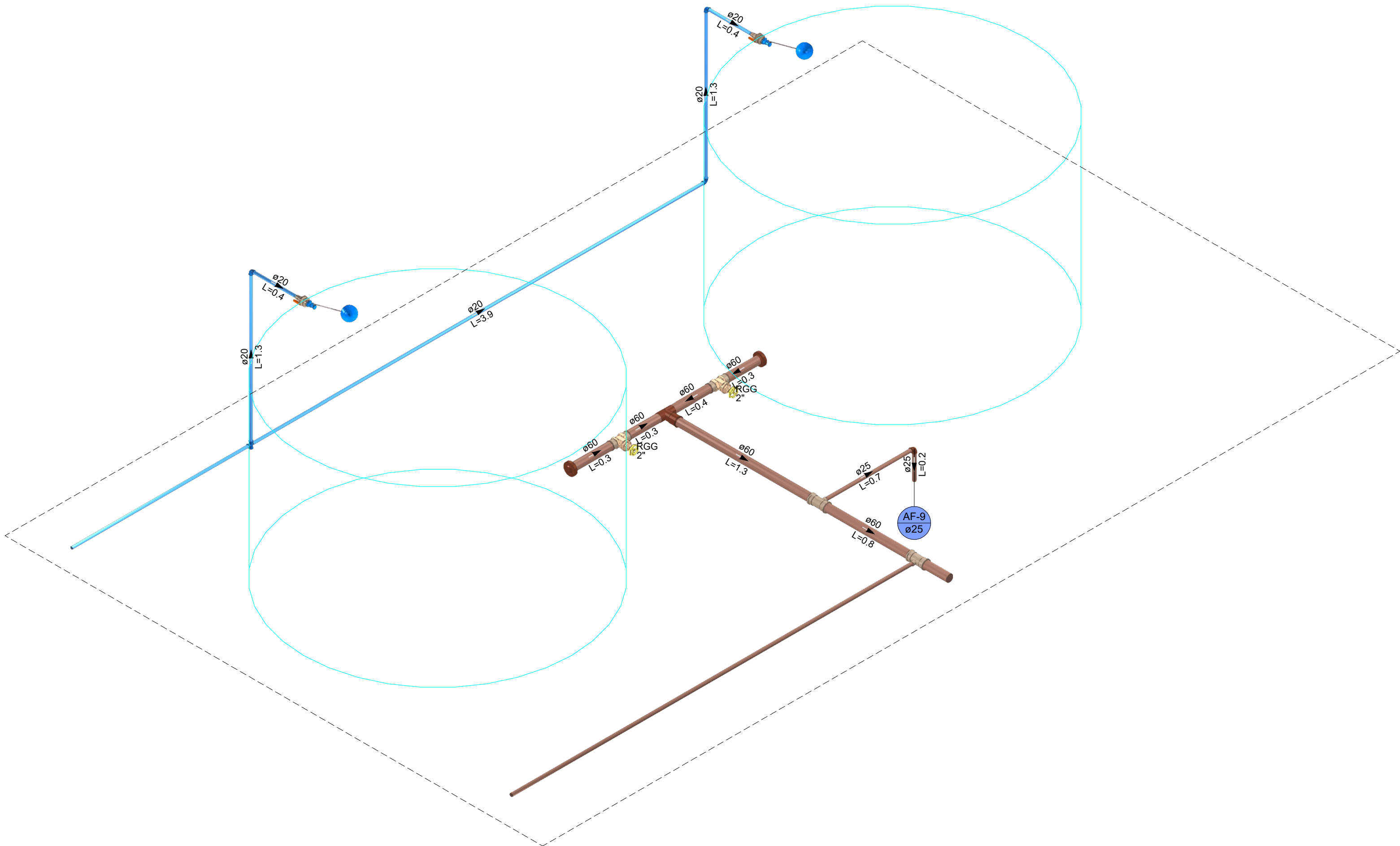
2 DETALHE H12 1:25
