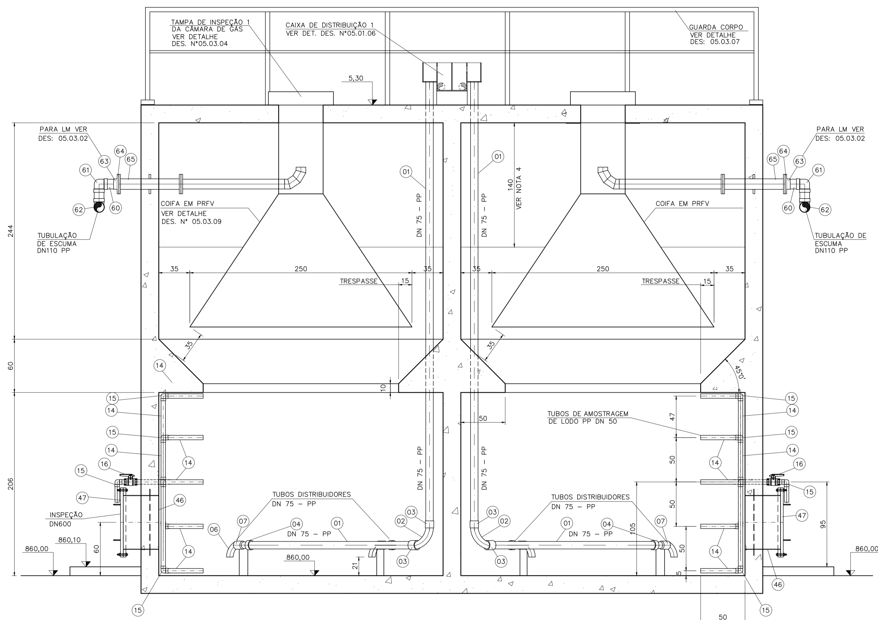
CORTE D-D ESC. 1:25
