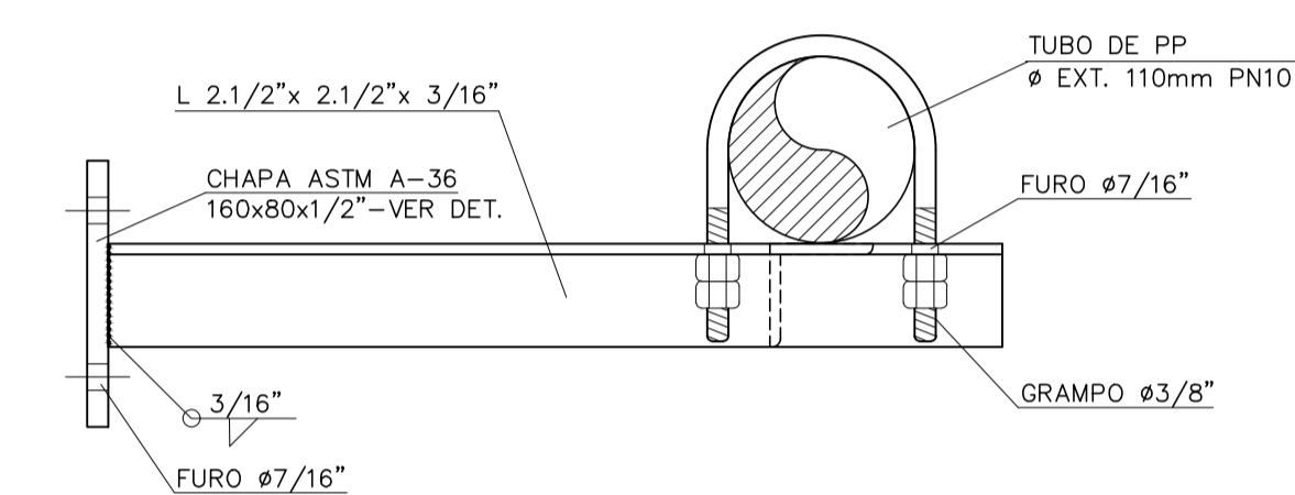
CORTE
