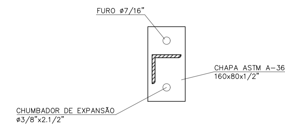
PLANTA
