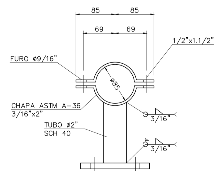
CORTE
