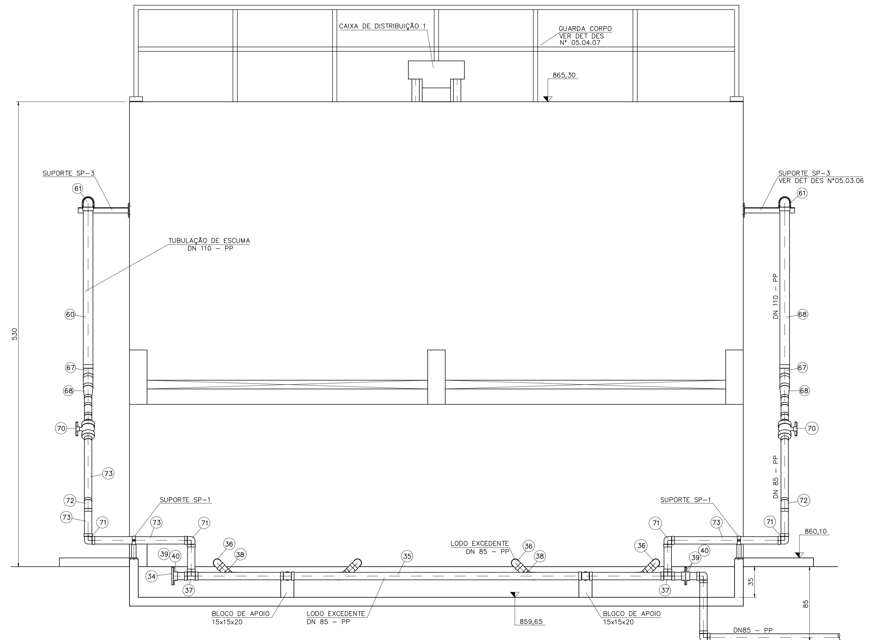
VISTA-02 ESC. 1:25
