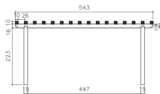
PERGOLADO - VISTA FRONTAL ESCALA 1:100
