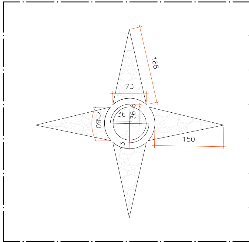
DETALHE ROSA DOS VENTOS ESCALA 1:50
