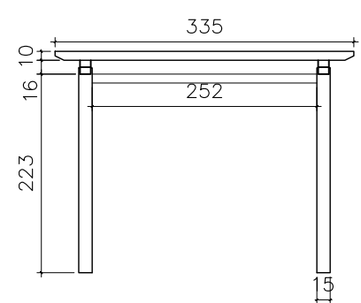
PERGOLADO - VISTA LATERAL
