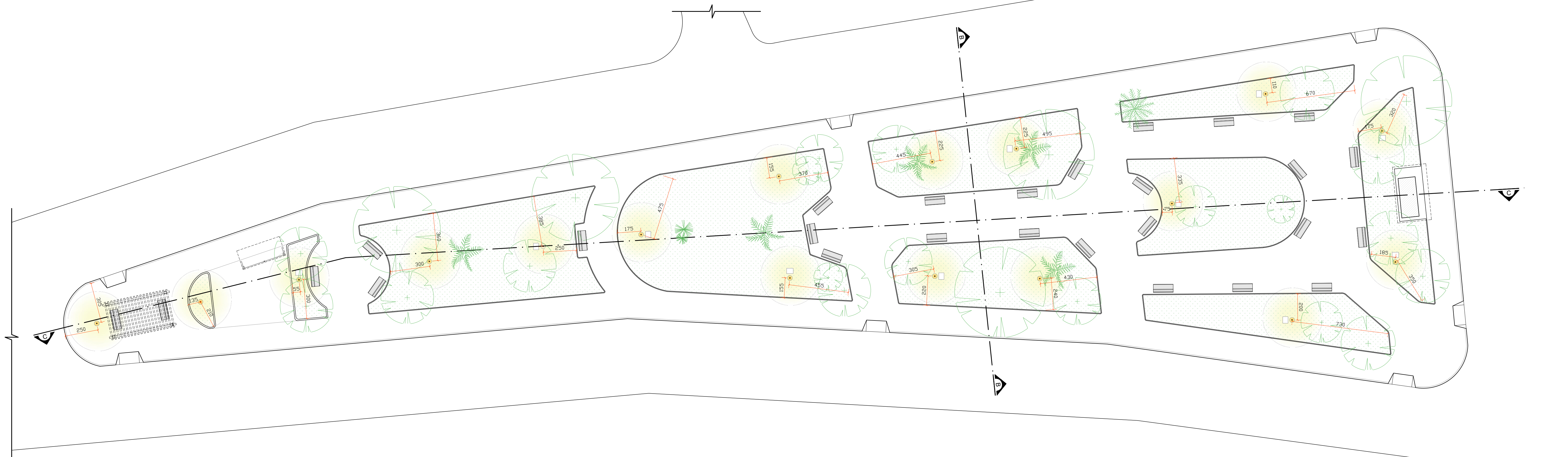
PLANTA DE ILUMINAÇÃO ESCALA 1:150
