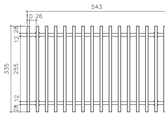
PERGOLADO - VISTA SUPERIOR
