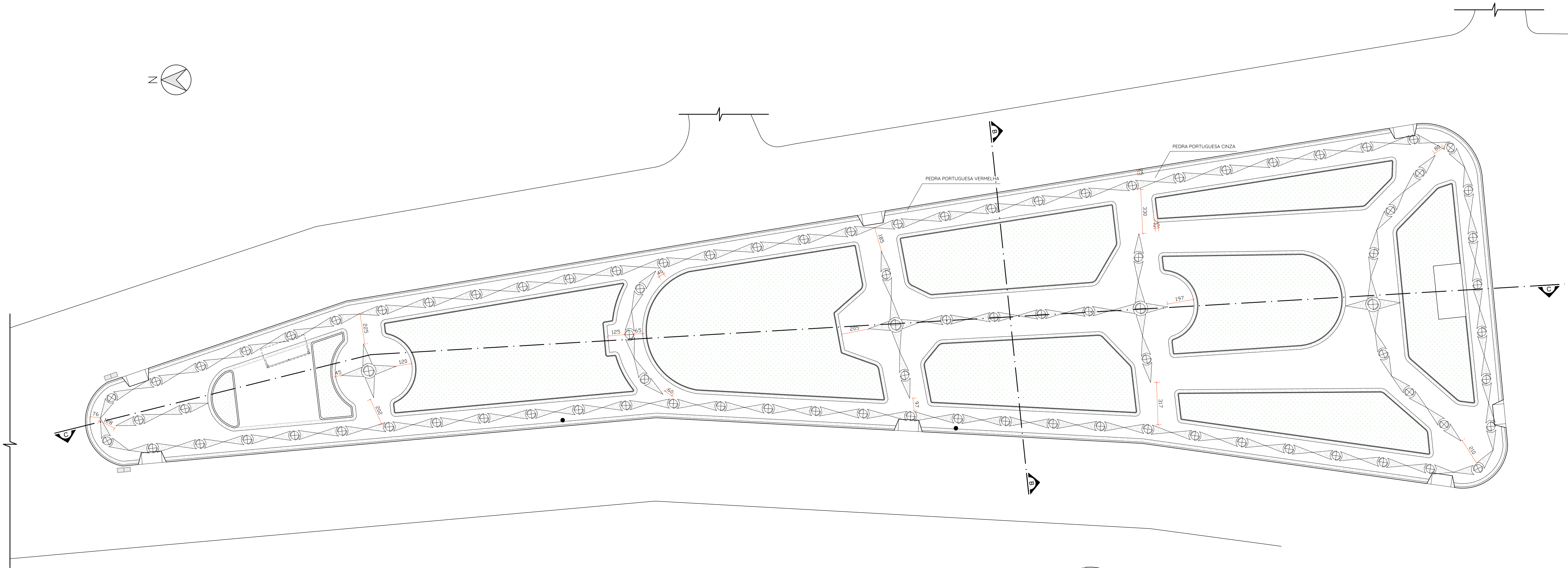
PLANTA DE PAGINAÇÃO DE PISO ESCALA 1:150
