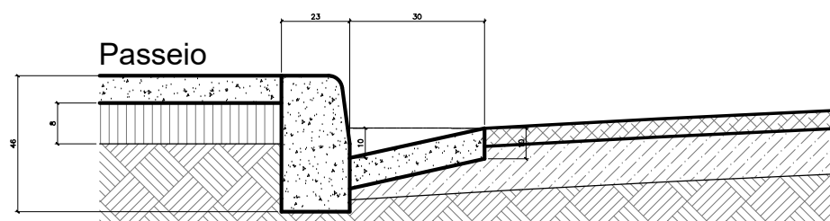
DETALHAMENTO DE SARJETA E MEIO-FIO Esc.: 1 : 15
