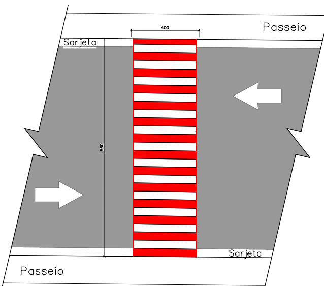
DETALHAMENTO FAIXA DE PEDESTRE sem escala
