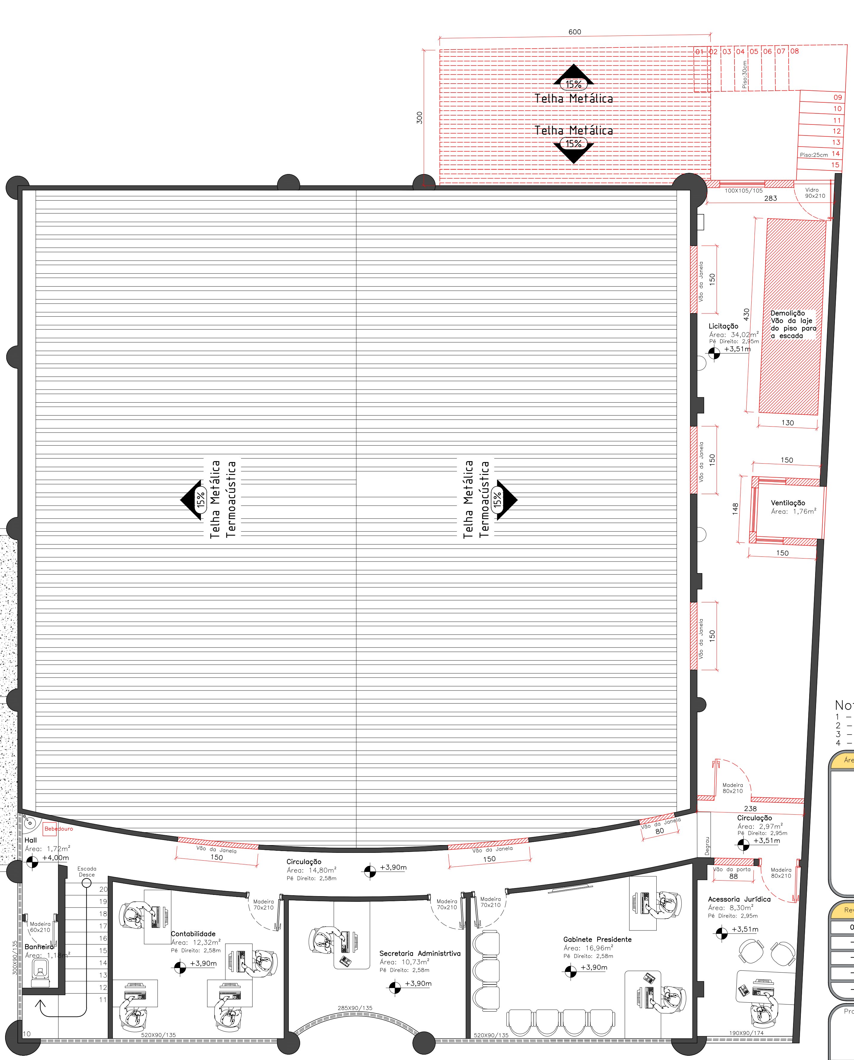
PLANTA DEMOLIÇÃO E REMOÇÃO NO PAVIMENTO SUPERIOR ESCALA 1:50
