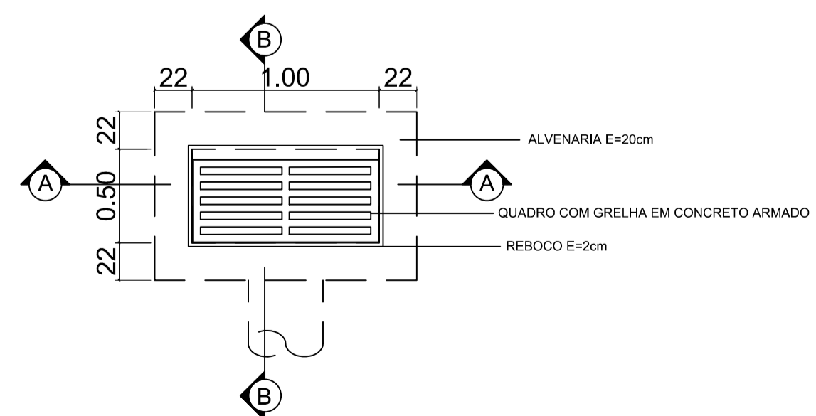
PLANTA
