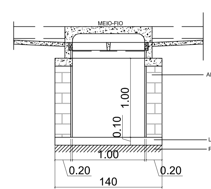
CORTE-AA
