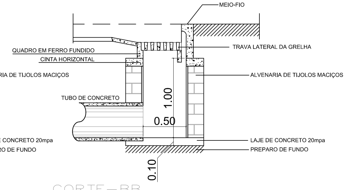
CORTE-BB
