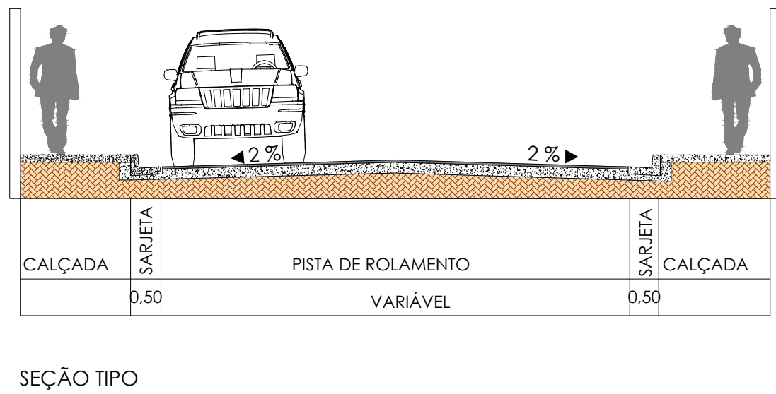
SEÇÃO TIPO
