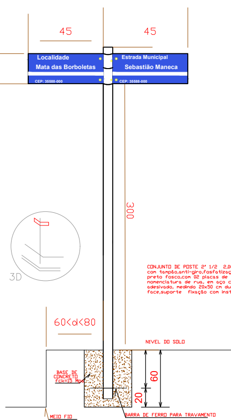
DETALHE PLACA ID - SEM ESCALA
