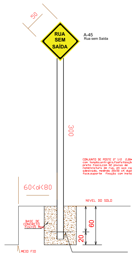
DETALHE PLACA A-45 - SEM ESCALA
