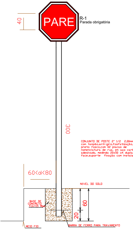
DETALHE PLACA R-1 - SEM ESCALA
