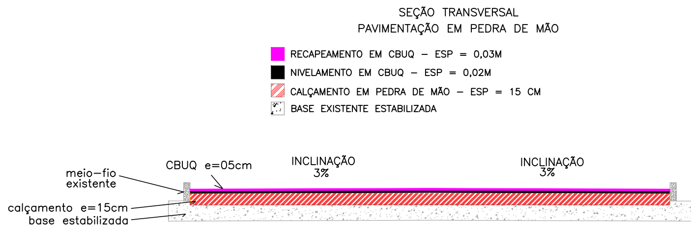
DETALHE SEÇÃO DA VIA - SEM ESCALA
