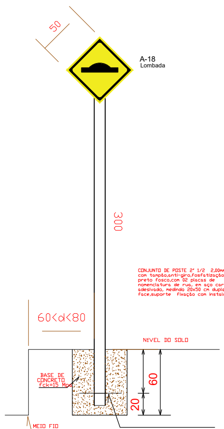
DETALHE PLACA A-18 - SEM ESCALA
