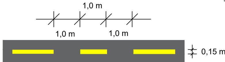
DETALHE SIN. HORIZONTAL - SEM ESCALA
