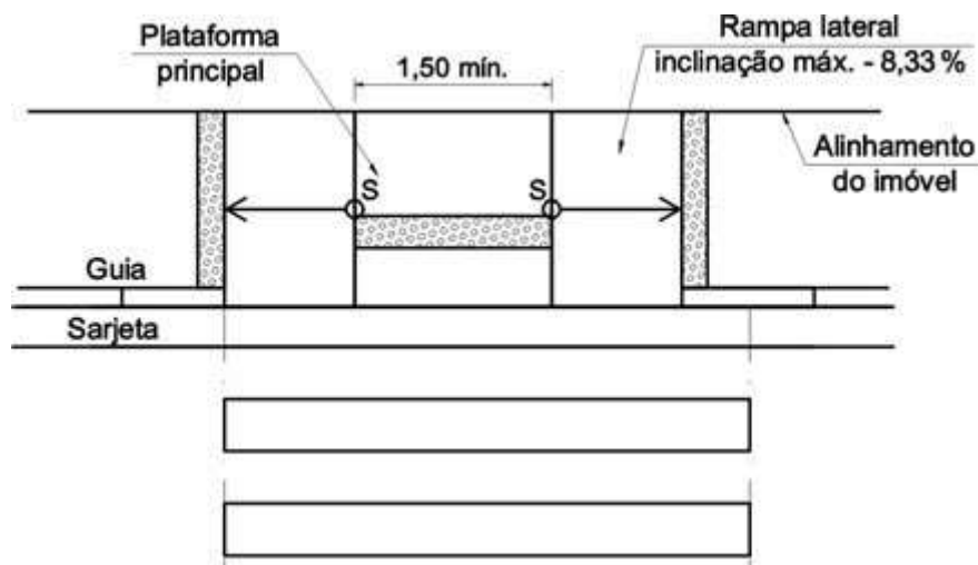
Figura 02: Imagem ilustrativa da rampa de acessibilidade nas calçadas.
