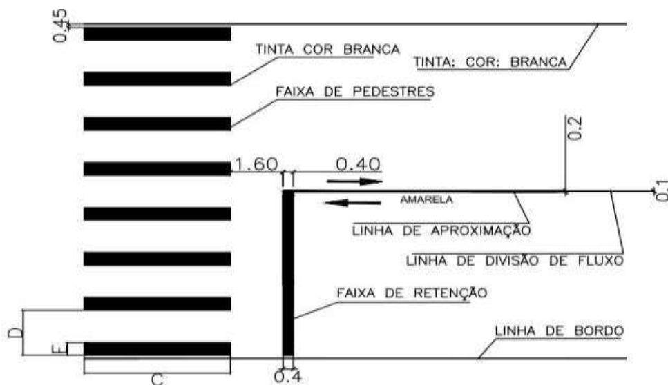
Figura 08: Detalhe complementar da faixa de pedestre
