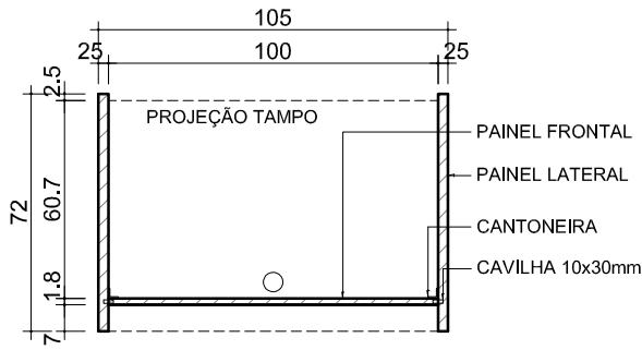
1 PLANTA BAIXA ESCALA 1/25
