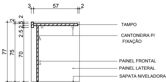
6 CORTE LONGITUDINAL ESCALA 1/25
