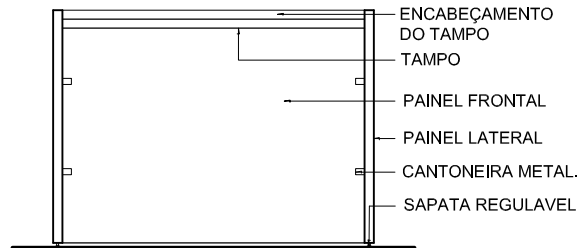
4 ELEVÇÃO POSTERIOR ESCALA 1/25
