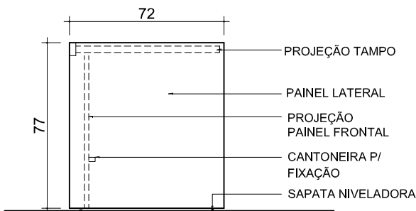
5 VISTA LATERAL ESCALA 1/25
