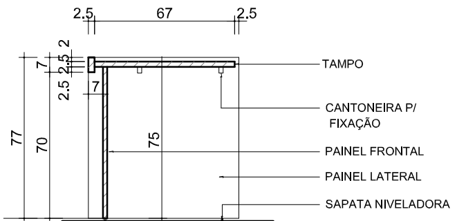
6 CORTE LONGITUDINAL ESCALA 1/25
