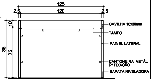
4 VISTA POSTERIOR ESCALA 1/25
