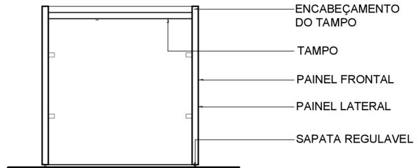
4 ELEVÇÃO POSTERIOR ESCALA 1/25
