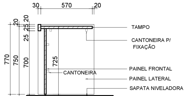
6 CORTE LONGITUDINAL ESCALA 1/25
