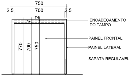
3 ELEVÇÃO FRONTAL ESCALA 1/25
