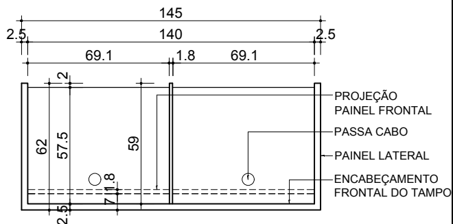
2 VISTA SUPERIOR ESCALA 1/25
