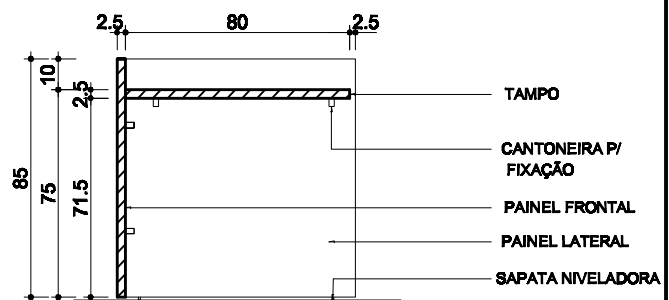
6 CORTE LONGITUDINAL ESCALA 1/25
