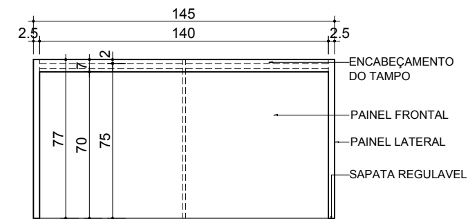
3 ELEVACÃO FRONTAL ESCALA 1/25
