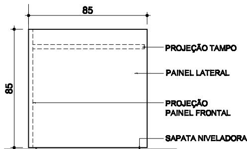
5 VISTA FRONTAL ESCALA 1/25
