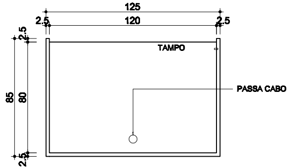
2 VISTA SUPERIOR ESCALA 1/25
