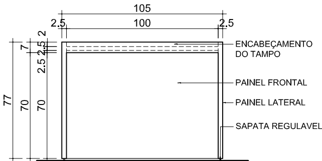
3 ELEVÇÃO FRONTAL ESCALA 1/25
