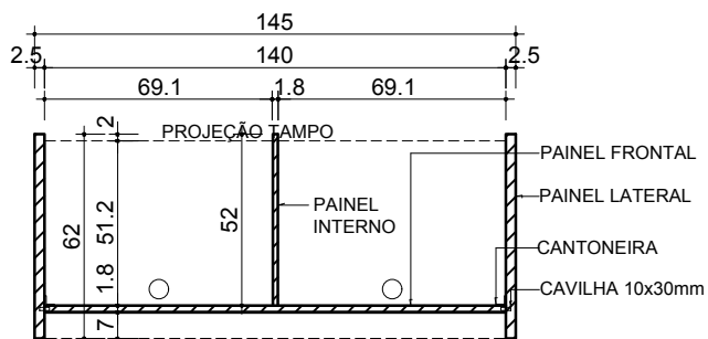
1 PLANTA BAIXA ESCALA 1/25
