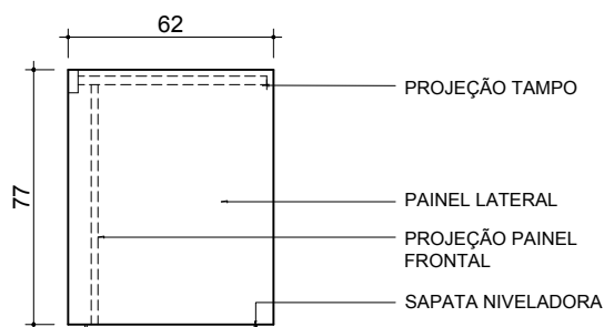
5 VISTA LATERAL ESCALA 1/25
