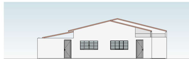
FACHADA FRONTAL ESC: 1 : 75
