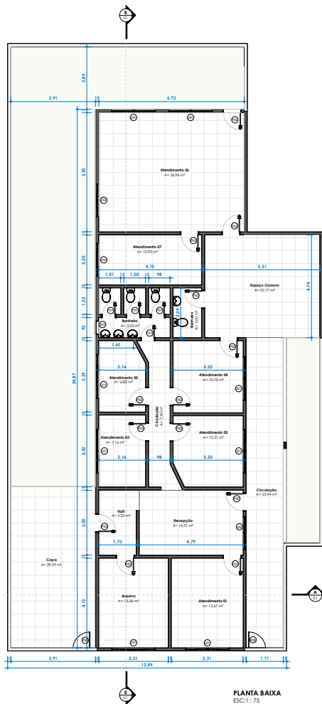
PLANTA BAIXA ESC: 1 : 75
