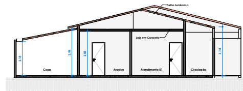
CORTE A-A ESC: 1 : 75
