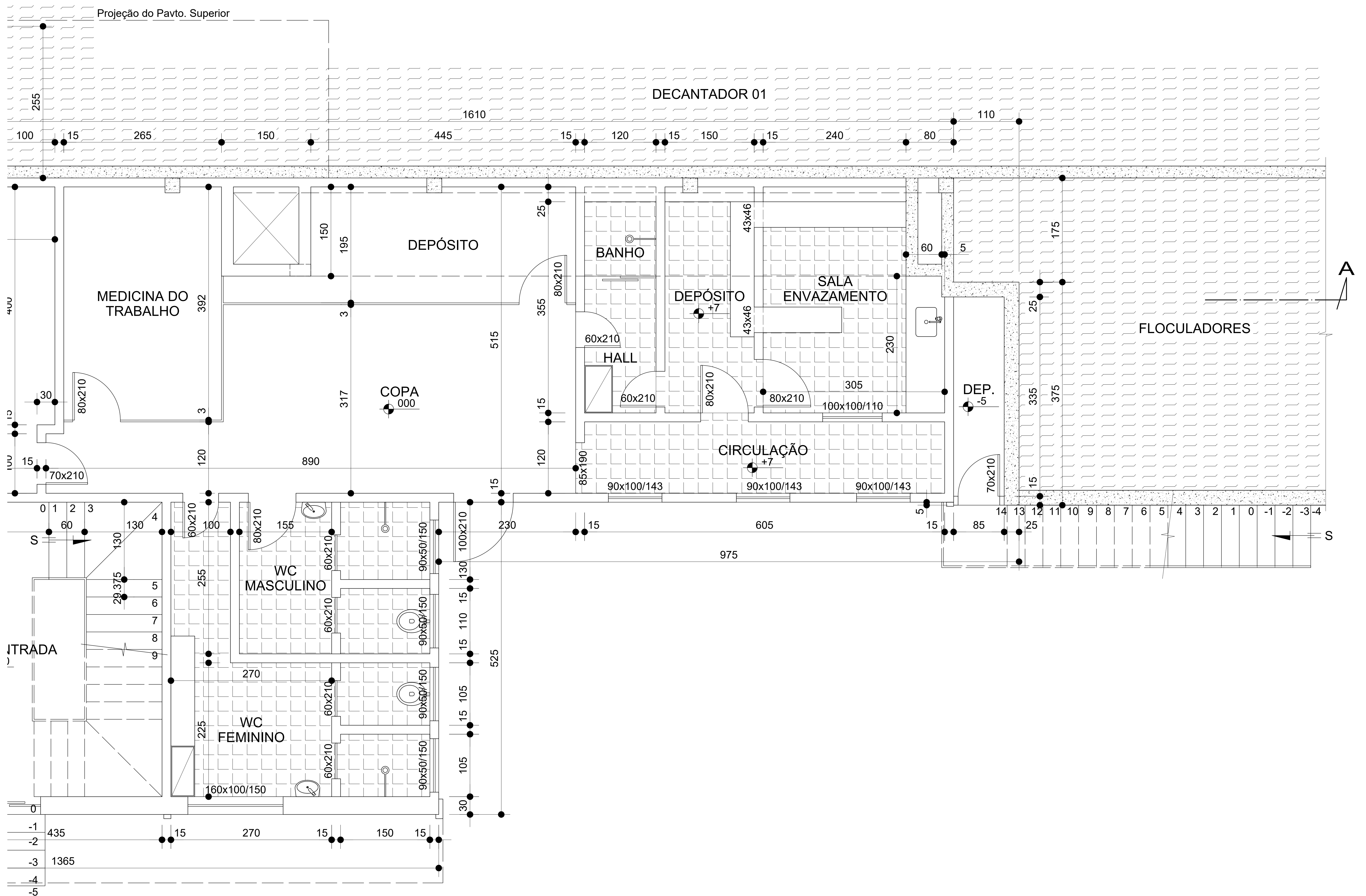
PLANTA BAIXA PAVTO. TÉRREO ESCALA 1:75
