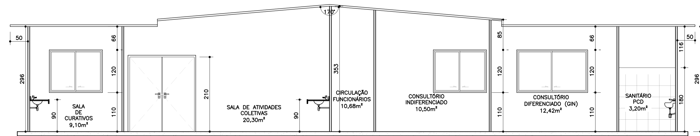
CORTE BB – MÓDULO SAÚDE- UBS esc: 1/100
