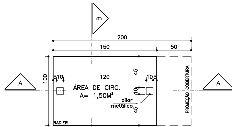
PLANTA BAIXA – ÁREA DE CIRCULAÇÃO esc 1/25
