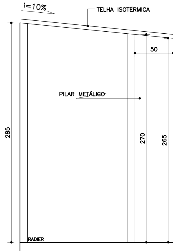
CORTE AA – ÁREA DE CIRCULAÇÃO esc 1/25
