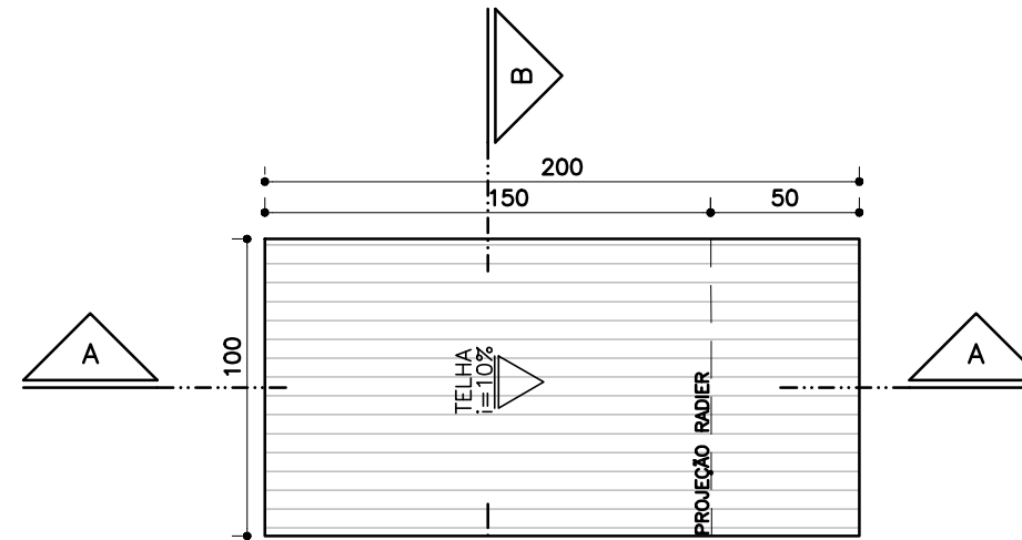
PLANTA COBERTURA – ÁREA DE CIRCULAÇÃO esc 1/25
