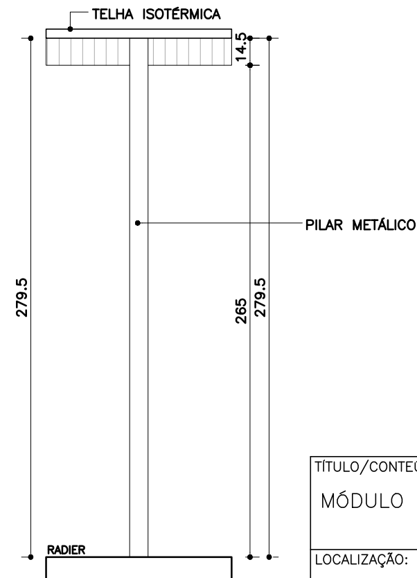
CORTE BB – ÁREA DE CIRCULAÇÃO esc 1/25
