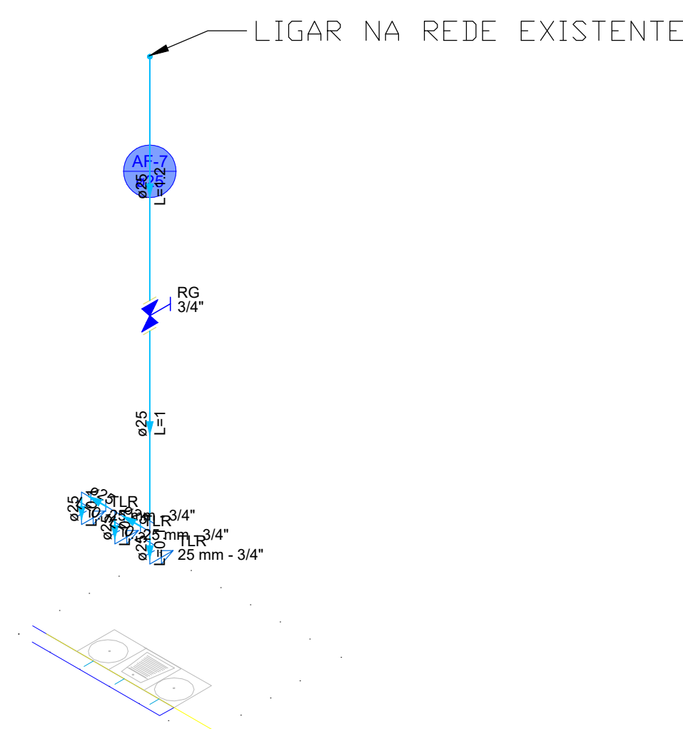
DETALHE HID-7 1:25
