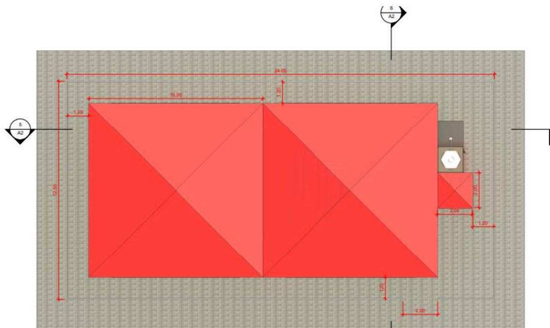
2 COBERTURA - PROJ 1 : 100
