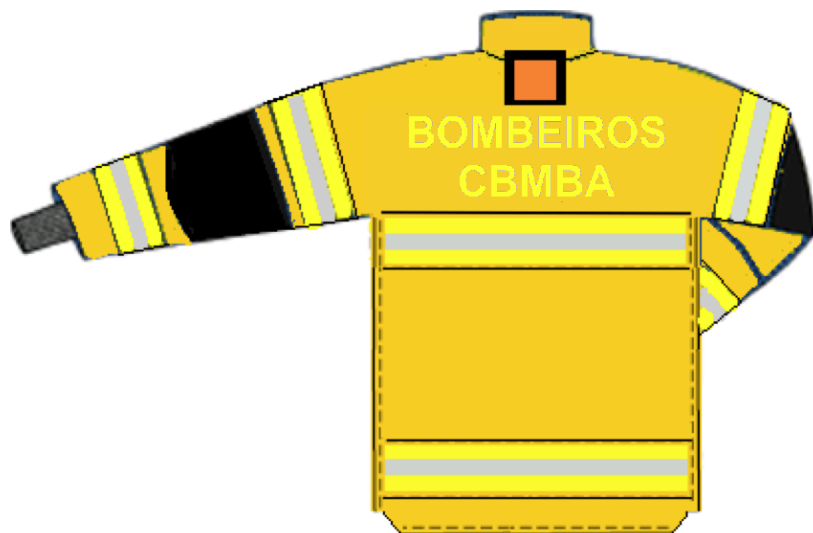
Fig. 5 - Vista dorsal do casaco de proteção e marcação da alça de salvamento
