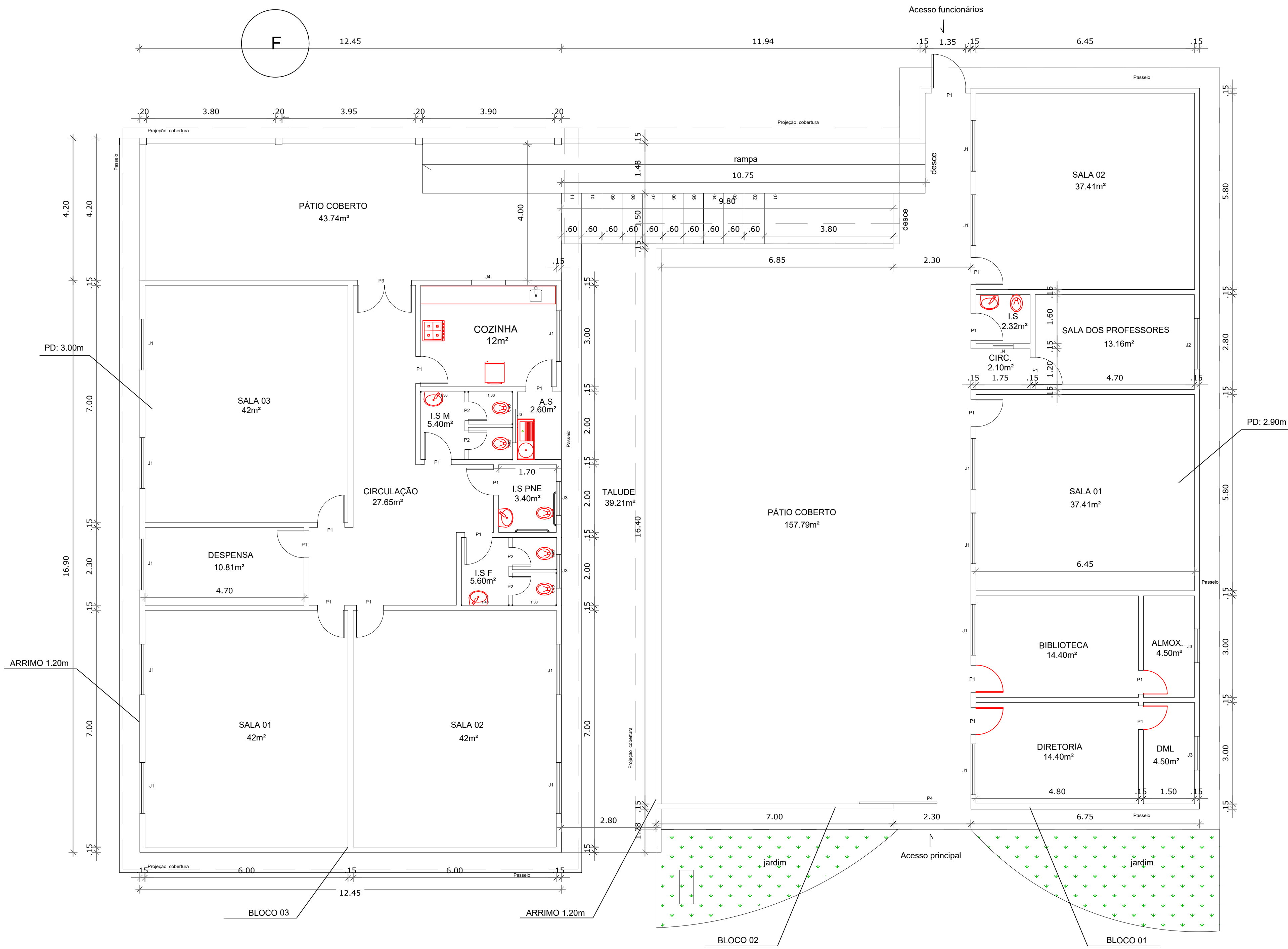
1 PLANTA - TÉRREO ESCALA 1/75
