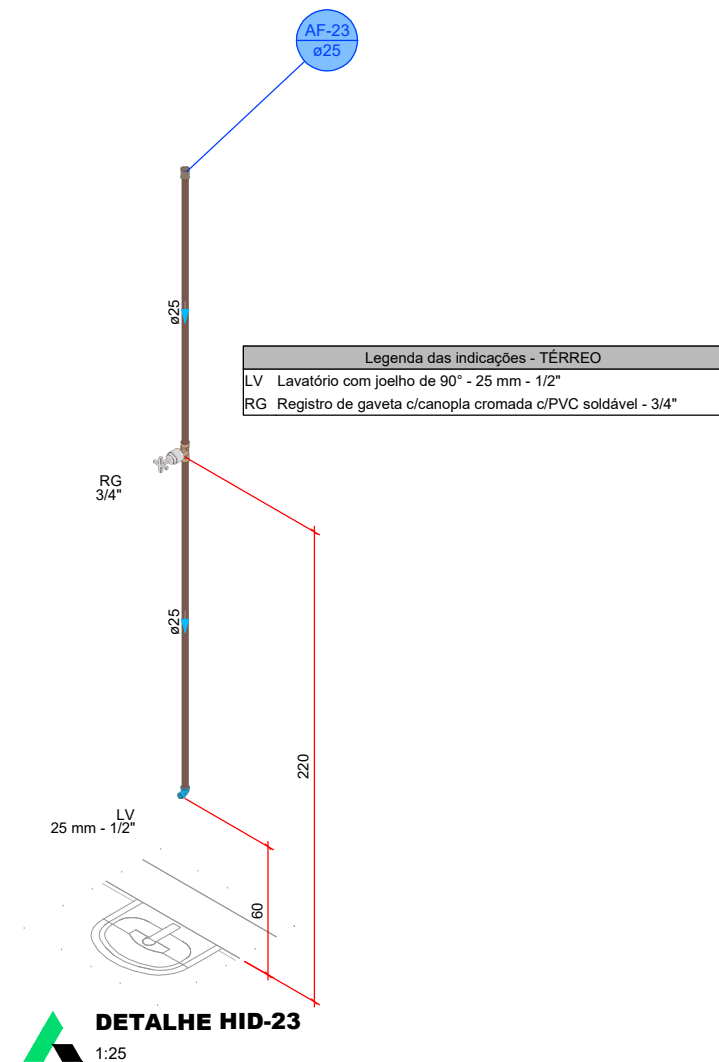
DETALHE HID-23
