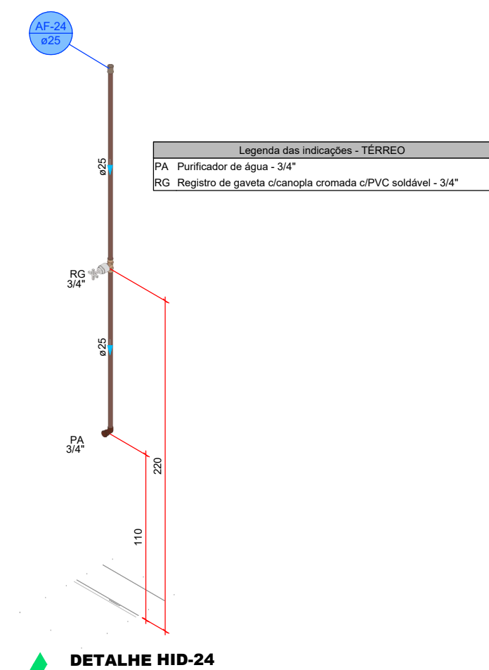
DETALHE HID-24
