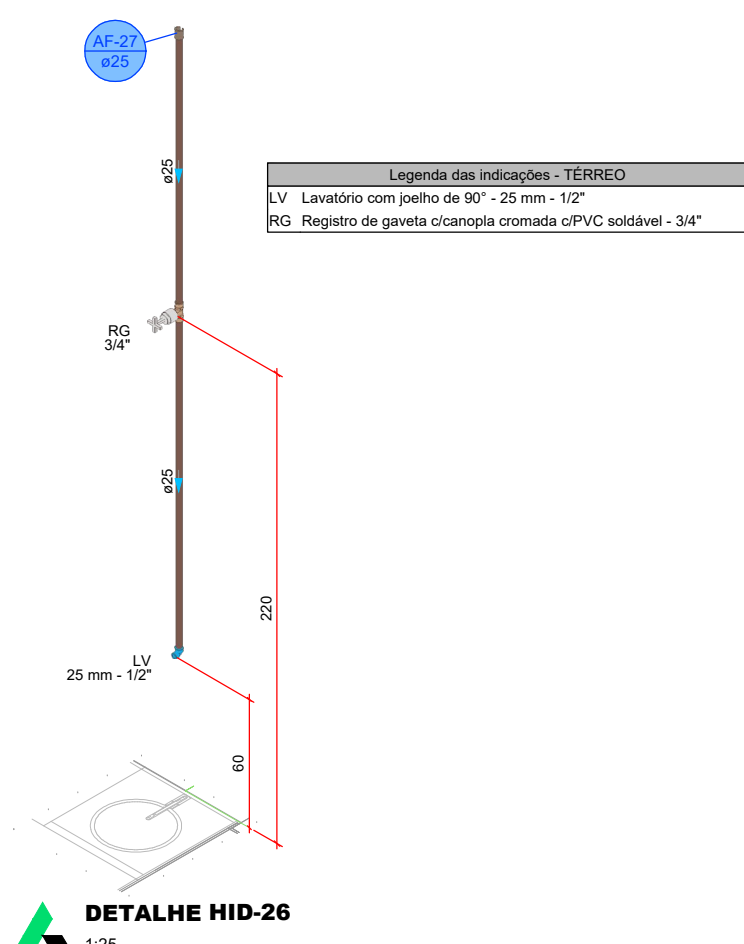
DETALHE HID-26
