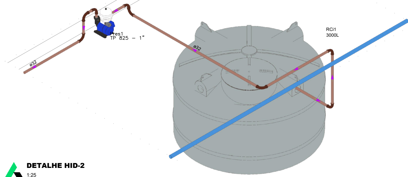
DETALHE HID-2 1:25
