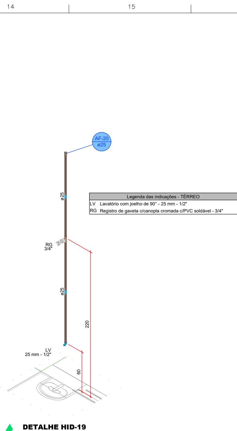
DETALHE HID-19
