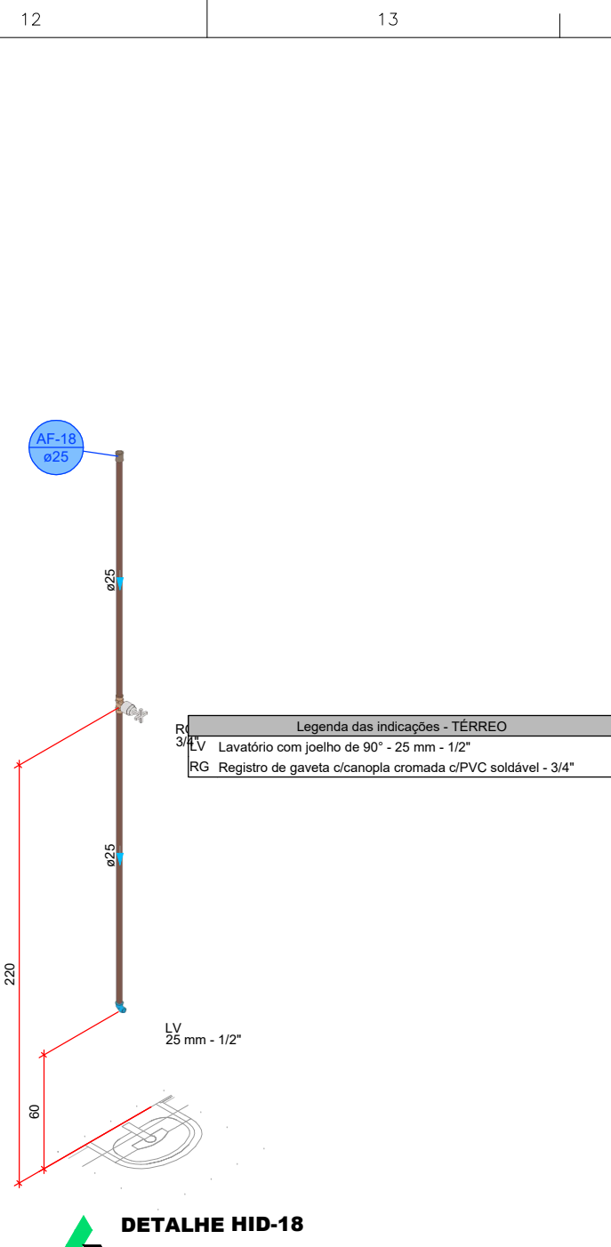
DETALHE HID-18
