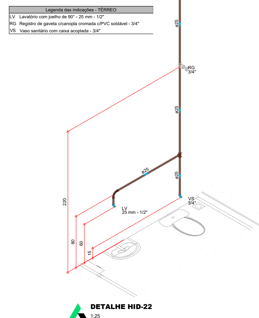
DETALHE HID-22
