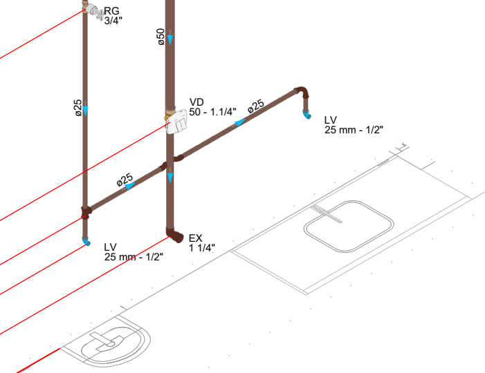
DETALHE HID-8 1:25
