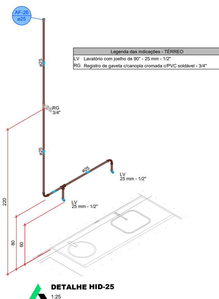
DETALHE HID-25
