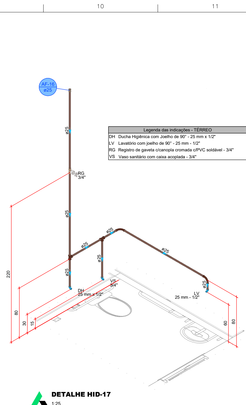
DETALHE HID-17
