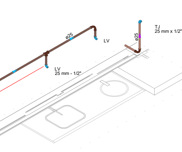
DETALHE HID-11 1:25
