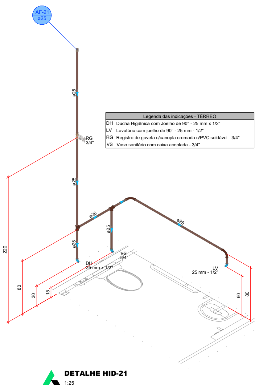
DETALHE HID-21
