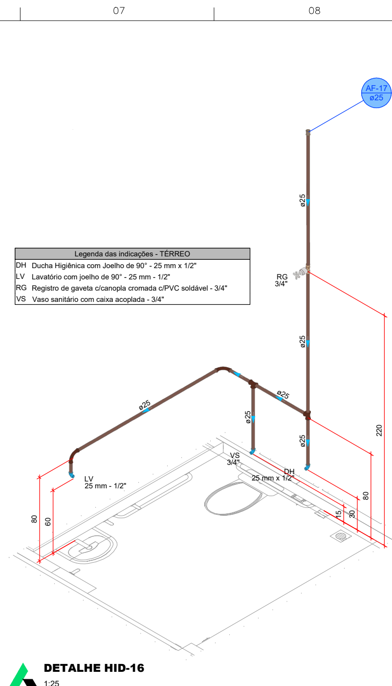
DETALHE HID-16
