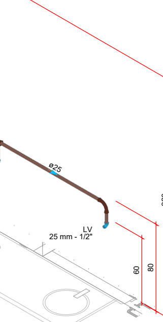
DETALHE HID-10 1:25
