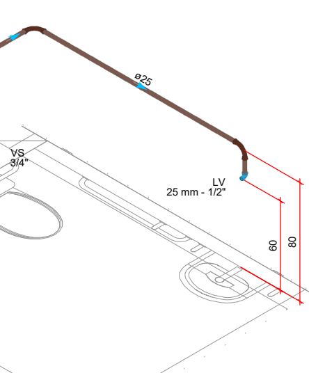
DETALHE HID-12 1:25
