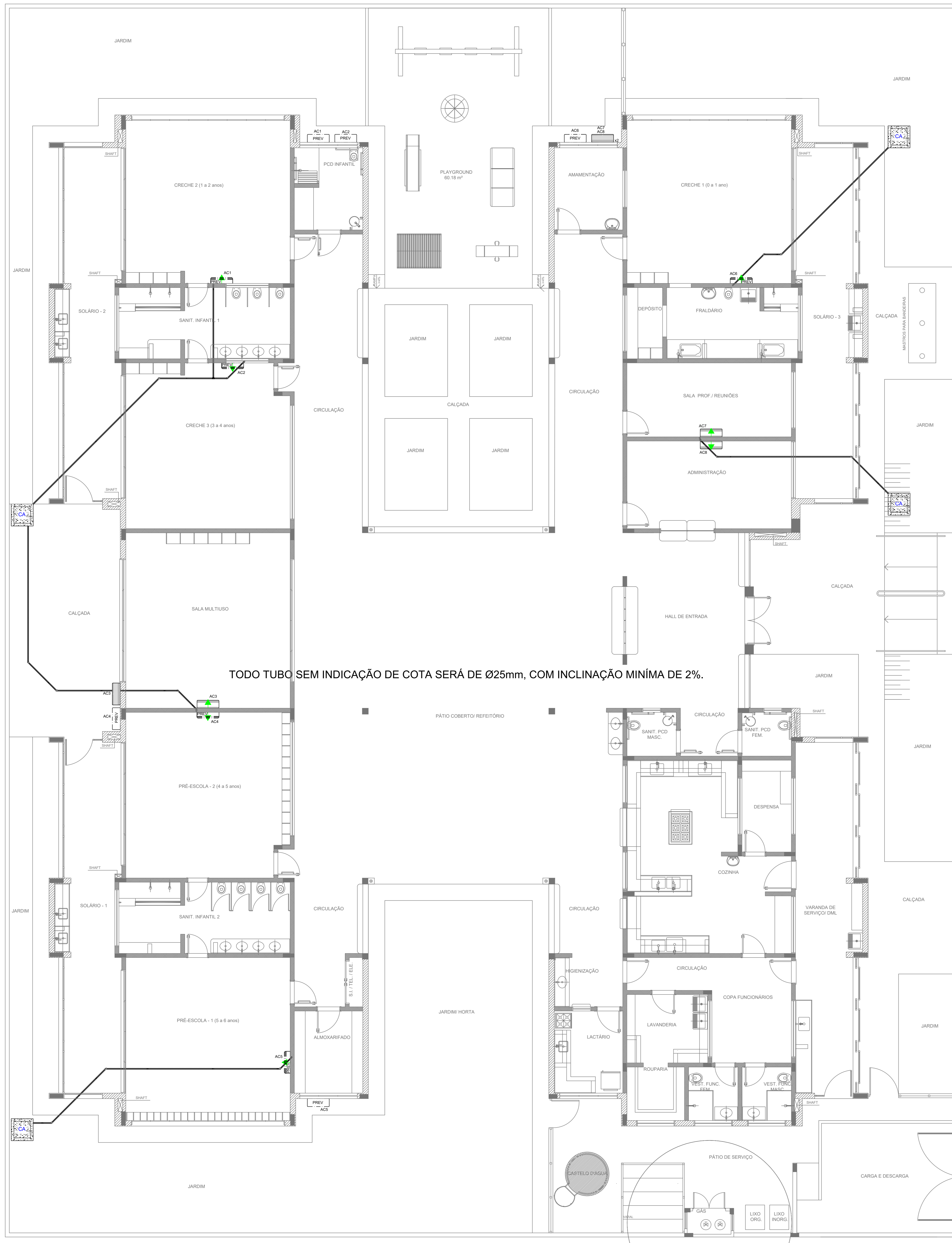
1 PLANTA BAIXA ESCALA 1/75
