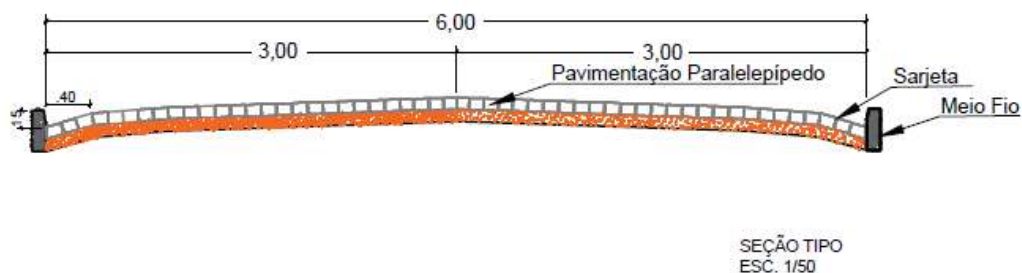
Fig. 04 - PAVIMENTAÇÃO SEÇÃO TIPO
