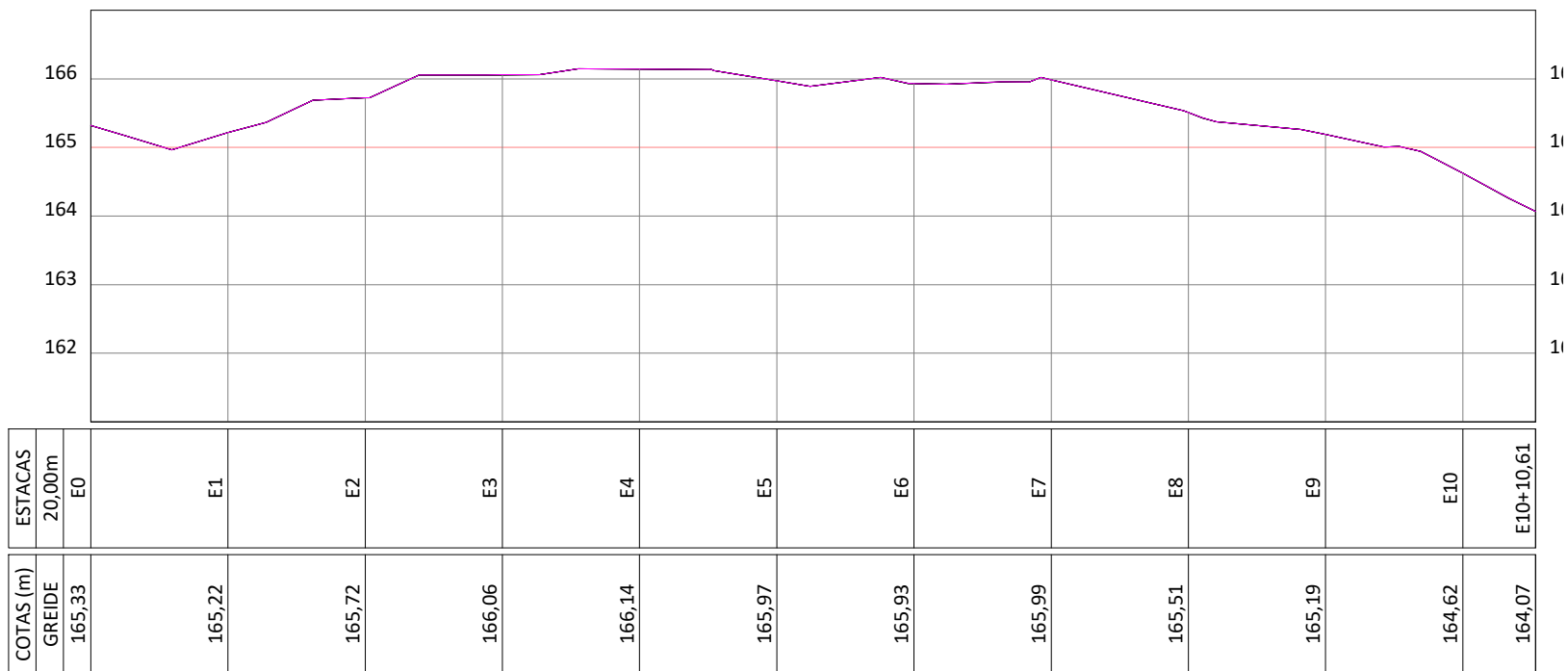
PERFIL LONGITUDINAL RUA PROJETADA 2 ESCALA VERTICAL 1/100 ESCALA HORIZONTAL 1/1000
