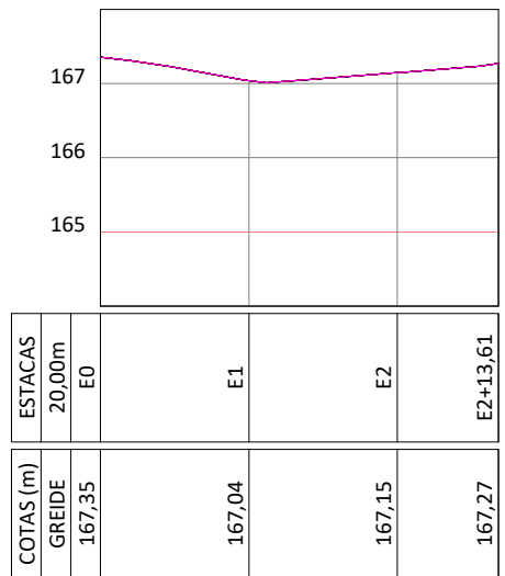
PERFIL LONGITUDINAL RUA PROJETADA 6 TRECHO 02 ESCALA VERTICAL 1/100 ESCALA HORIZONTAL 1/1000
