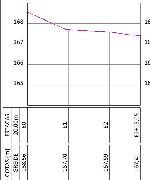
PERFIL LONGITUDINAL RUA PROJETADA 6 TRECHO 01 ESCALA VERTICAL 1/100 ESCALA HORIZONTAL 1/1000
