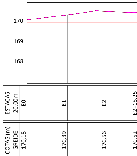
PERFIL LONGITUDINAL RUA PROJETADA 7 TRECHO 02 ESCALA VERTICAL 1/100 ESCALA HORIZONTAL 1/1000
