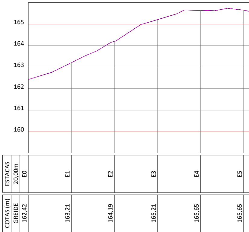
PERFIL LONGITUDINAL RUA PROJETADA 8 ESCALA VERTICAL 1/100 ESCALA HORIZONTAL 1/1000
