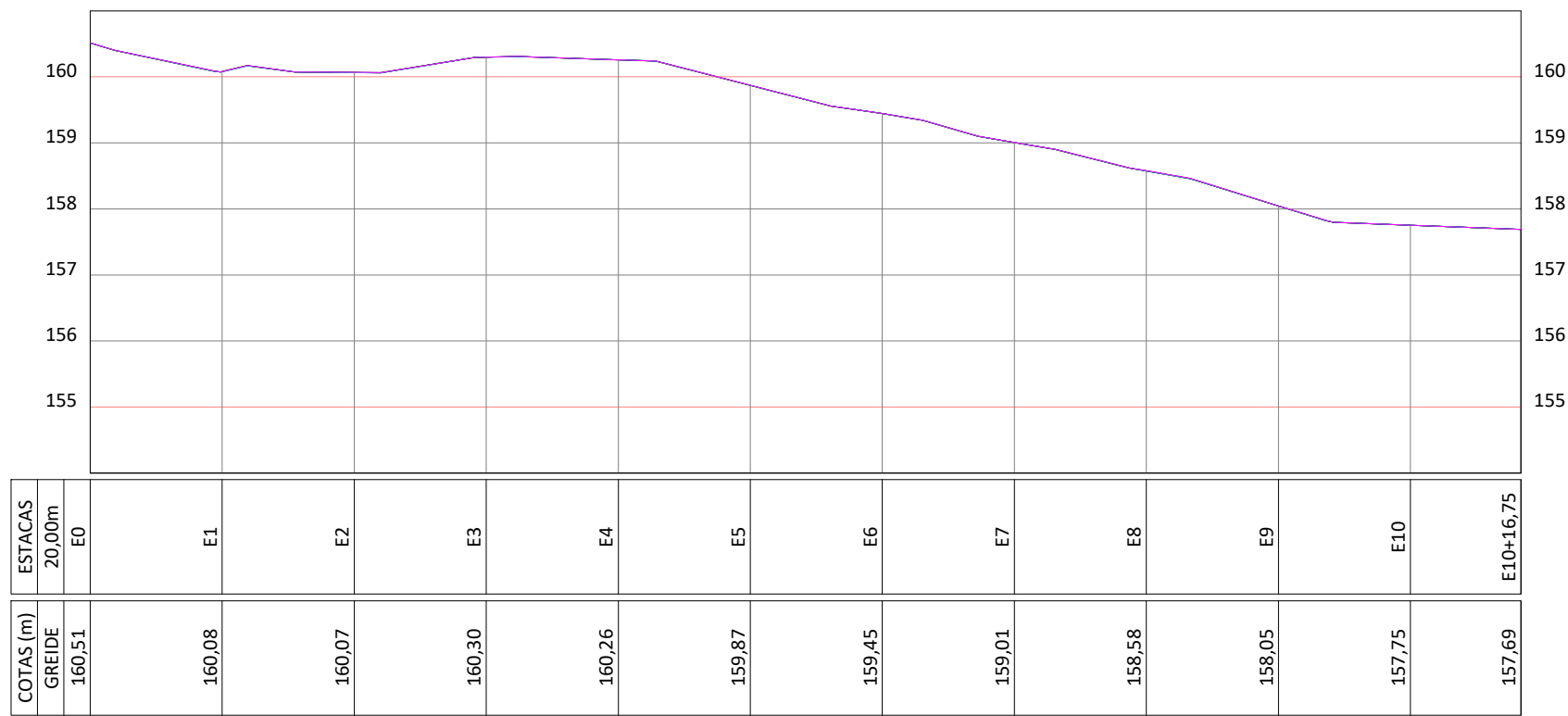
PERFIL LONGITUDINAL RUA PROJETADA 4 ESCALA VERTICAL 1/100 ESCALA HORIZONTAL 1/1000
