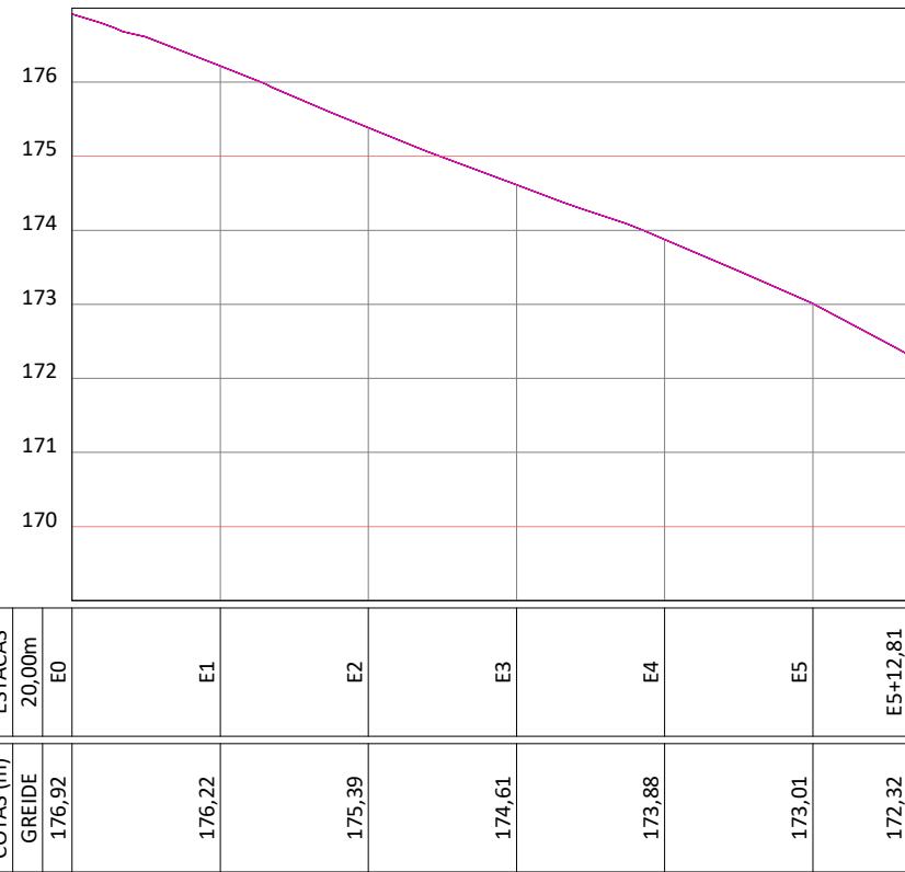
PERFIL LONGITUDINAL RUA JORDANIO TRECHO 01 ESCALA VERTICAL 1/100 ESCALA HORIZONTAL 1/1000
