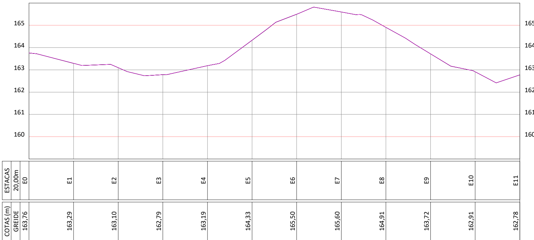
PERFIL LONGITUDINAL RUA PROJETADA 2 ESCALA VERTICAL 1/100 ESCALA HORIZONTAL 1/1000
