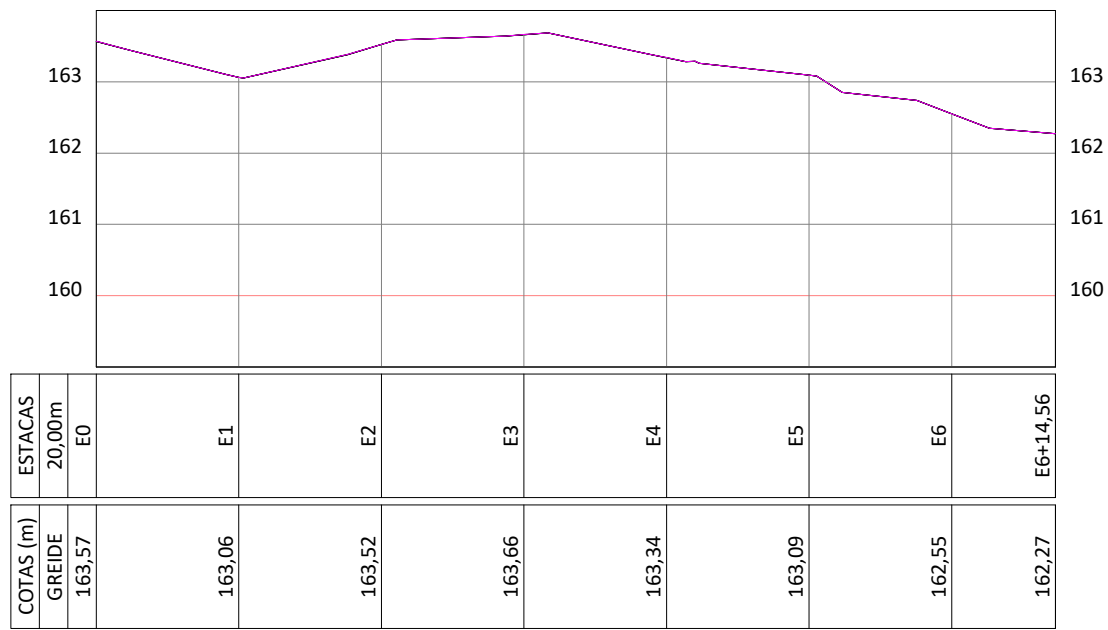
PERFIL LONGITUDINAL AV. PETRONIO PORTELA ESCALA VERTICAL 1/100 ESCALA HORIZONTAL 1/1000
