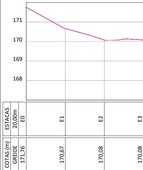
PERFIL LONGITUDINAL RUA PROJETADA 7 TRECHO 01 ESCALA VERTICAL 1/100 ESCALA HORIZONTAL 1/1000
