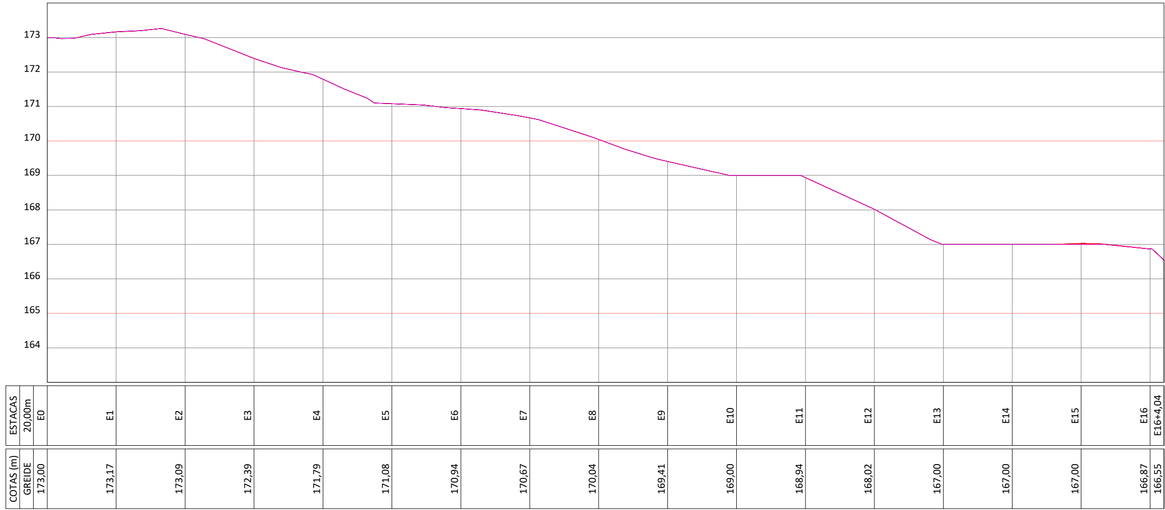
PERFIL LONGITUDINAL RUA PROJETADA 5 ESCALA VERTICAL 1/100 ESCALA HORIZONTAL 1/1000
