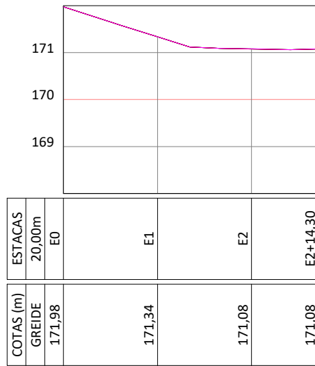
PERFIL LONGITUDINAL RUA JORDANIO TRECHO 02 ESCALA VERTICAL 1/100 ESCALA HORIZONTAL 1/1000
