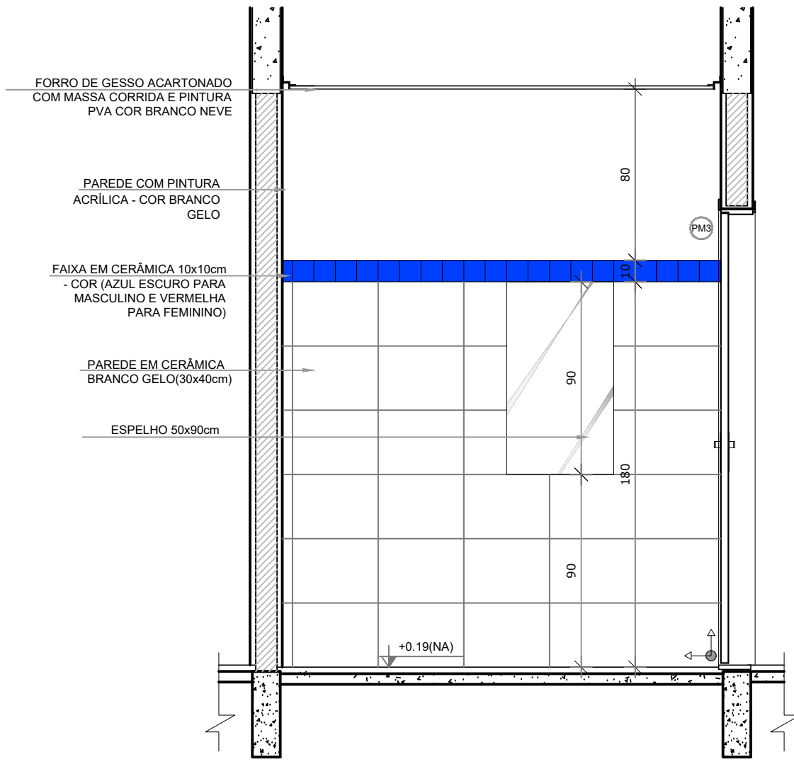
VISTA 4
