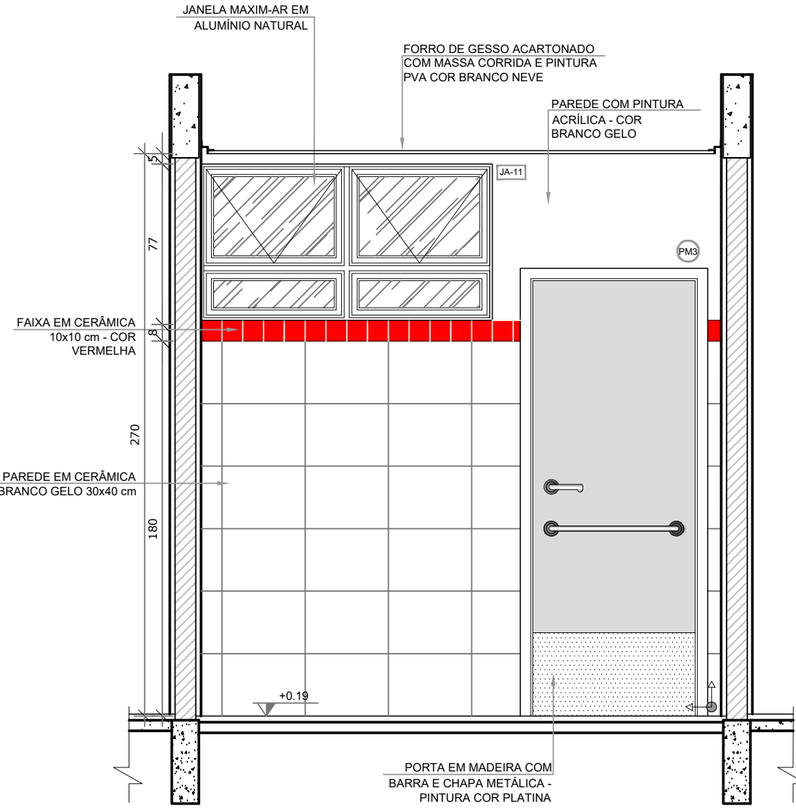
VISTA 4
