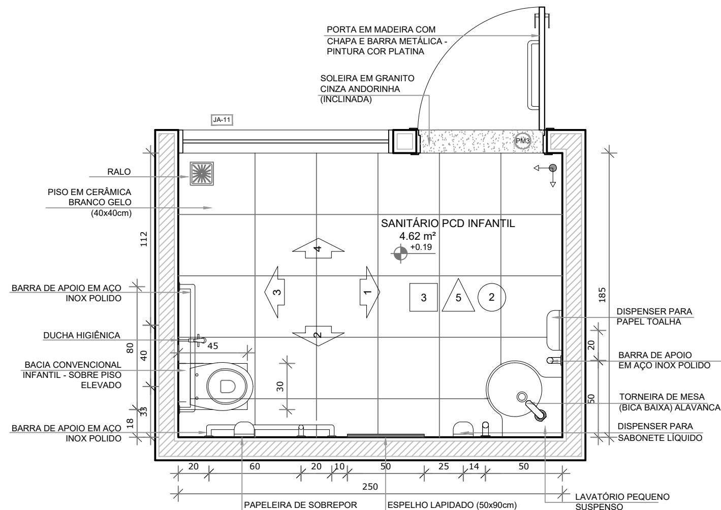
PLANTA BAIXA
