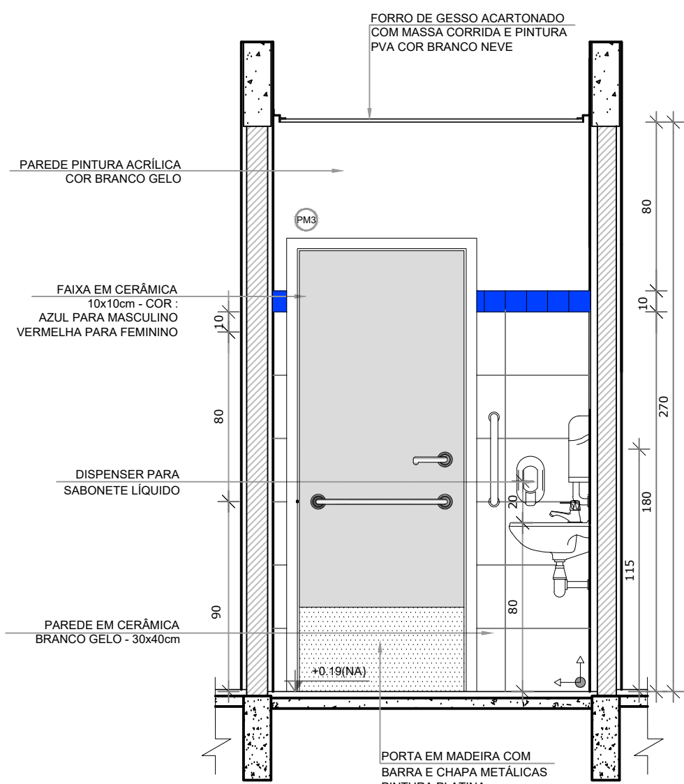
VISTA 1
