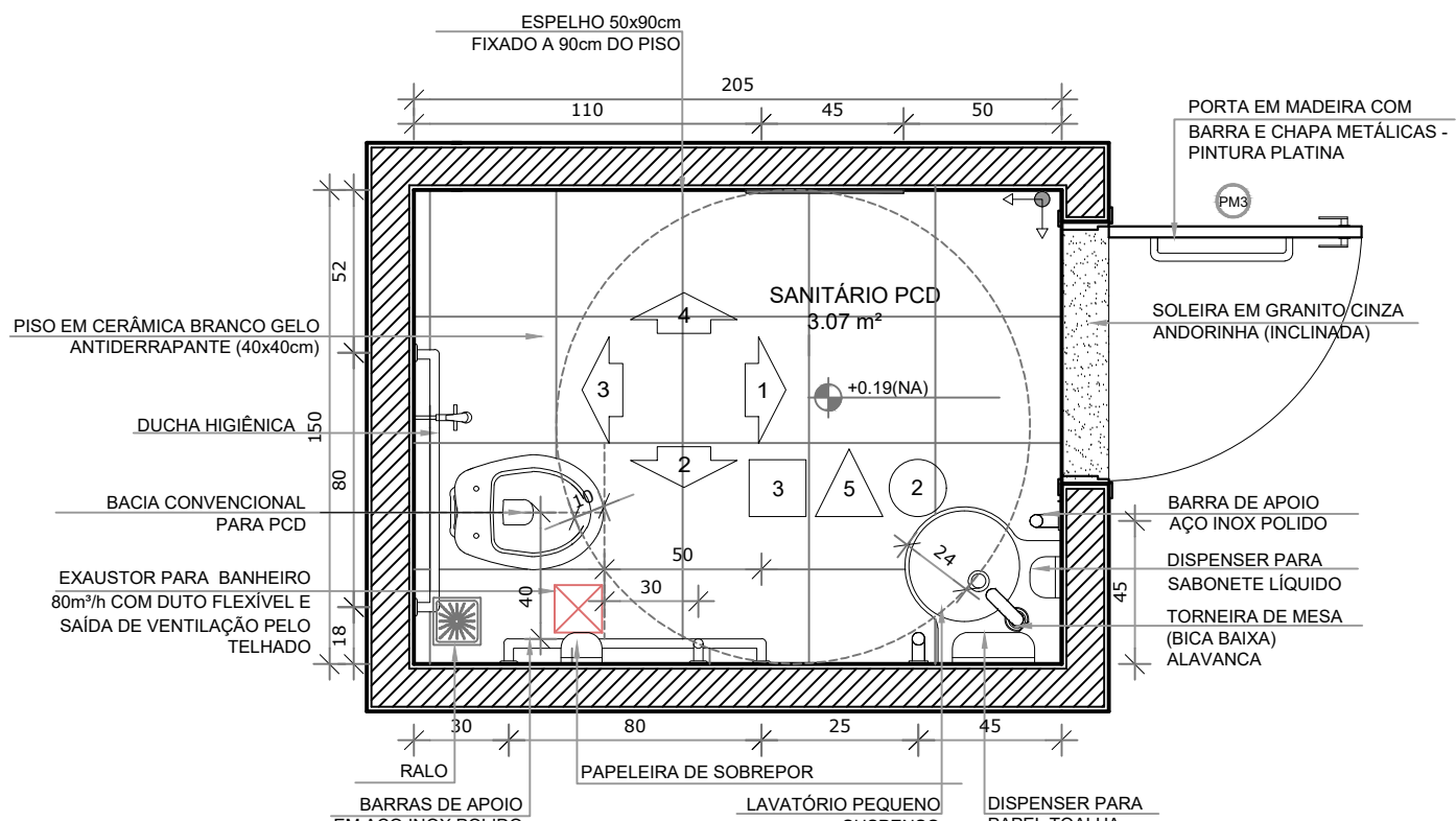
PLANTA BAIXA
