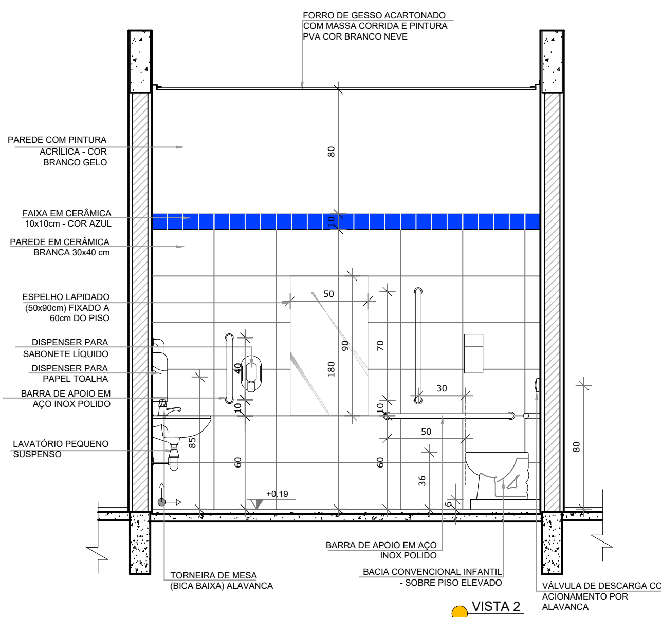
VISTA 2
