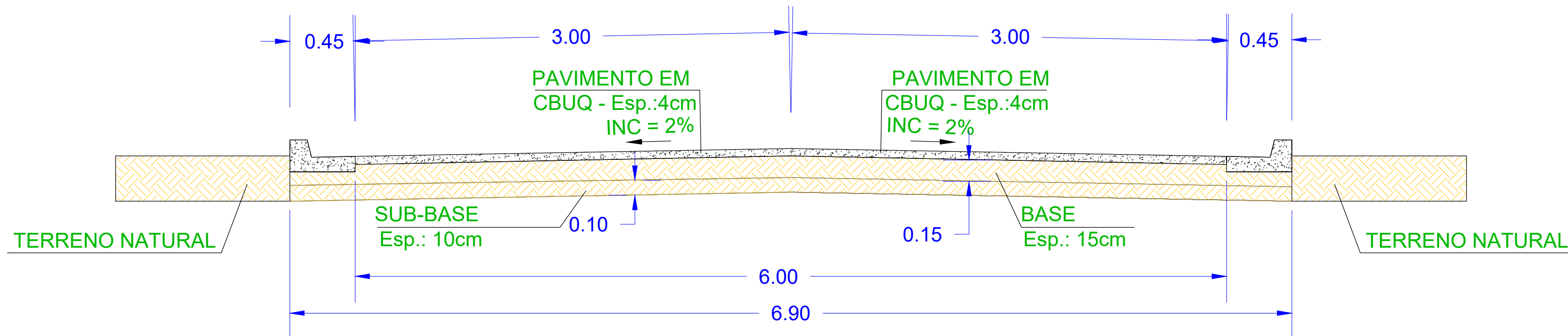
SEÇÃO TRANSVERSAL TÍPICA DA PAV. DA ESTRADA VICINAL BACABAL Estacas de 0,00 até 4+16,19 Estacas de 10+3,81 até 35,00 Esc.: 1/ 25
