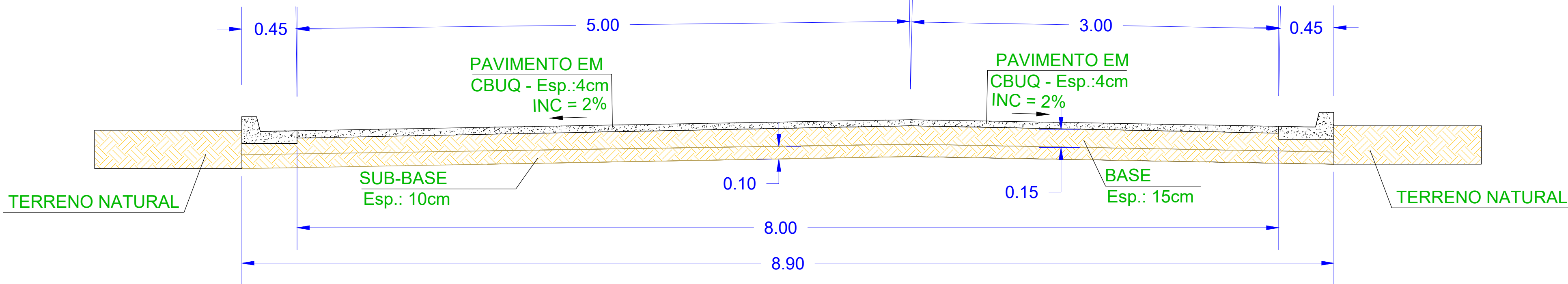
SEÇÃO TRANSVERSAL COM SUPERLARGURA DE FAIXA DA PAV. DA ESTRADA VICINAL BACABAL - ESTACA 8 Esc.: 1/ 25
