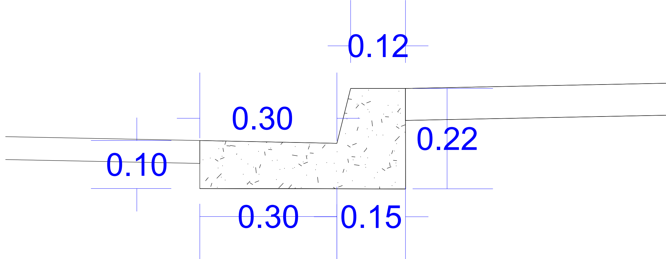
DETALHE - MEIO FIO E SARJETA CONJUGADA Esc.: 1/ 5
