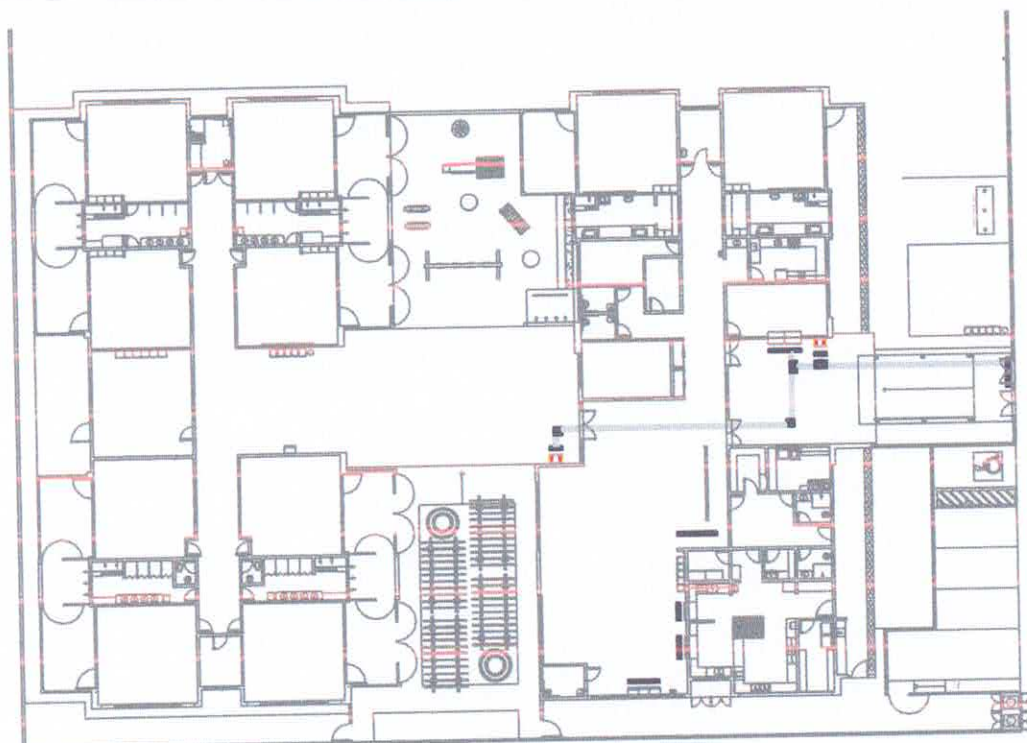
PLANTA DE SINALIZAÇÃO
