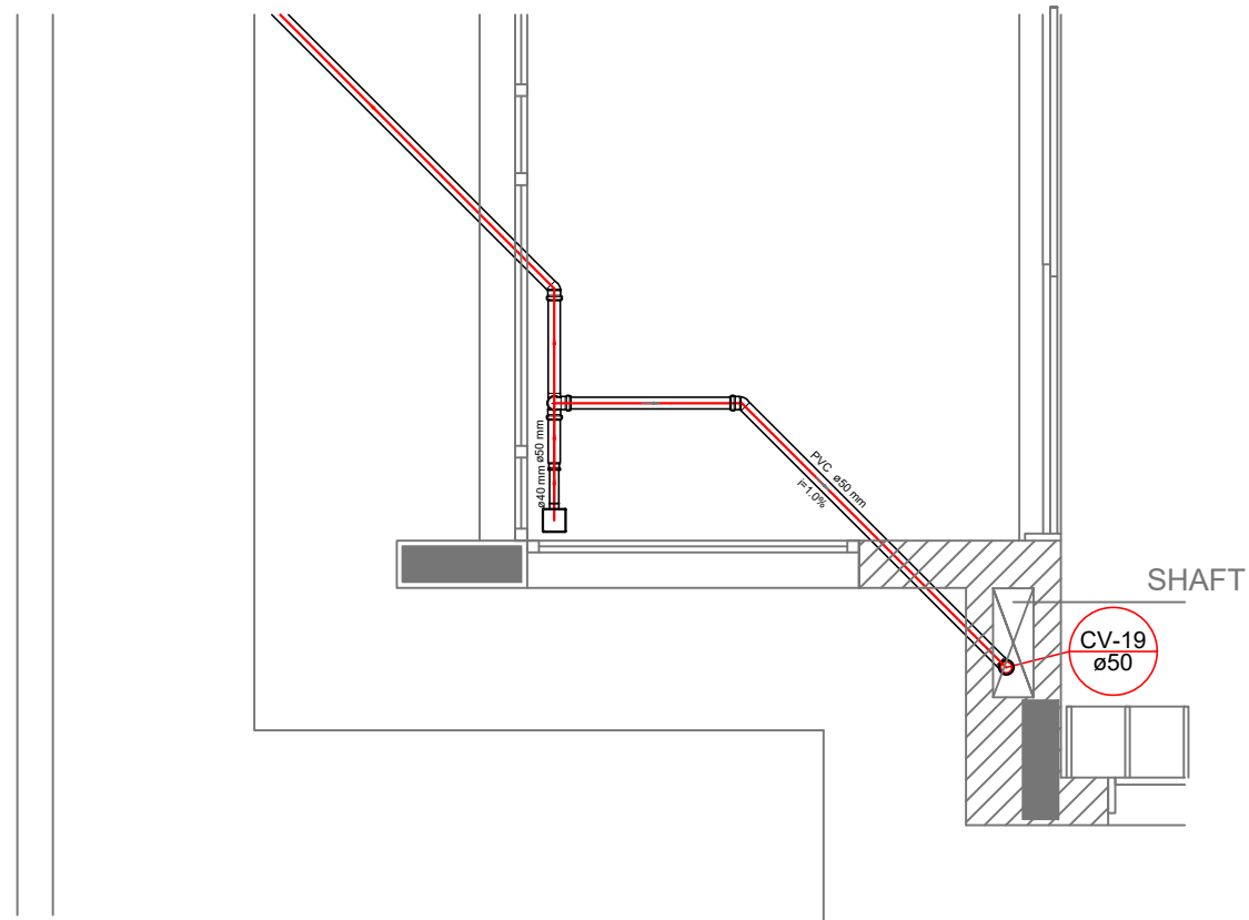
Detalhe S13 escala 1:25
