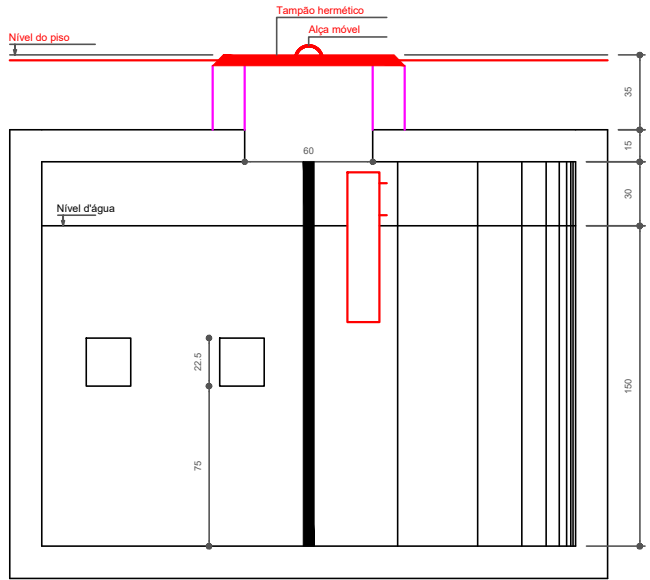
TANQUE SÉPTICO CORTE - ESC. 1:25
