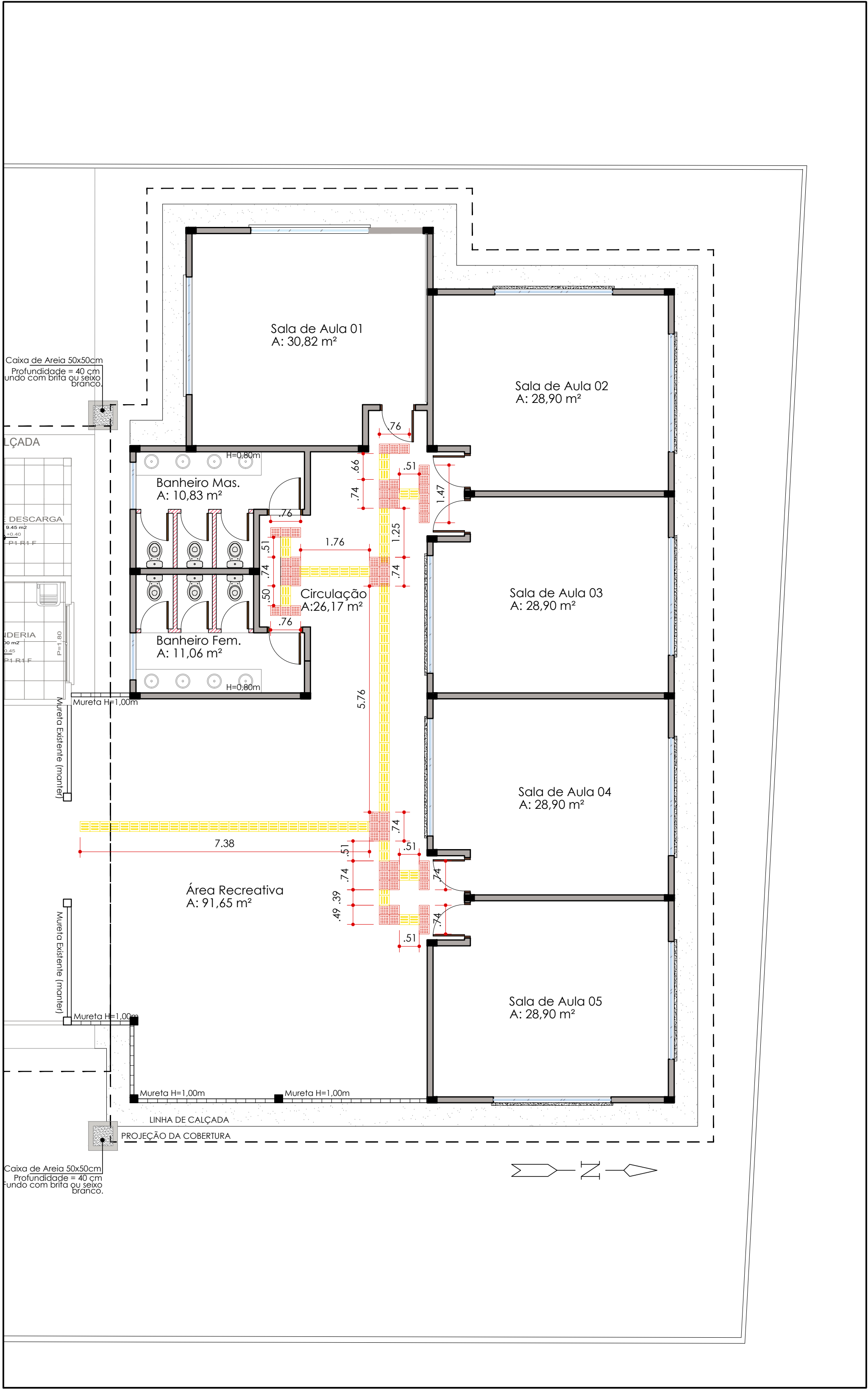
2 PLANTA DE ACESSIBILIDADE AMPLIAÇÃO ESCALA: 1:75 A: 340,69 M²
