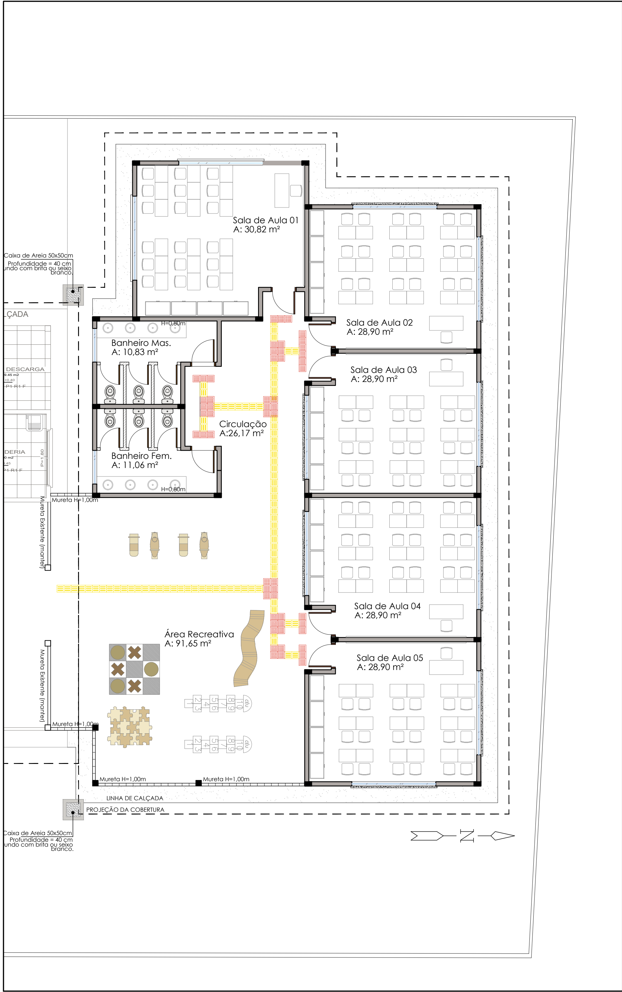
1 PLANTA LAYOUT AMPLIAÇÃO ESCALA: 1:75 A: 340,69 M²
