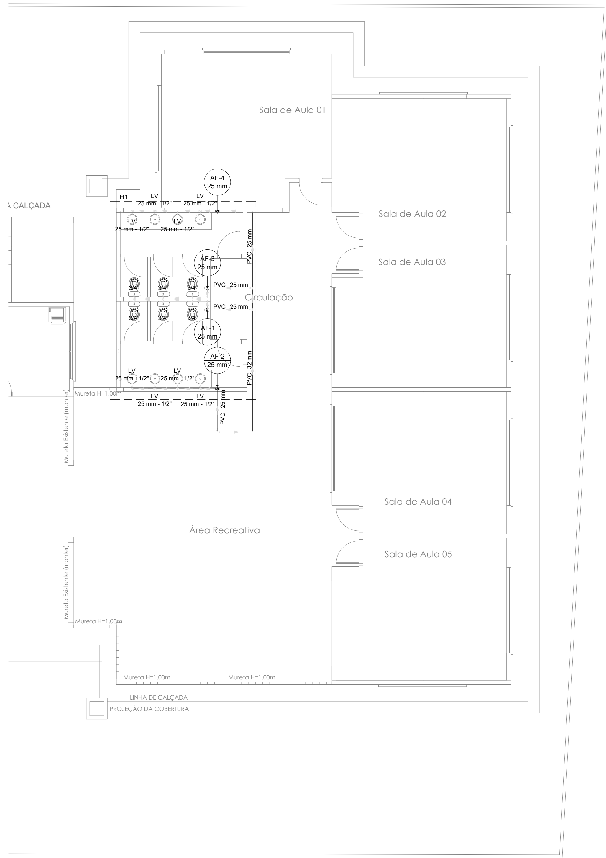
2 PLANTA DE ÁGUA FRIA ESCALA: 1:75 A: 340,69 M²
