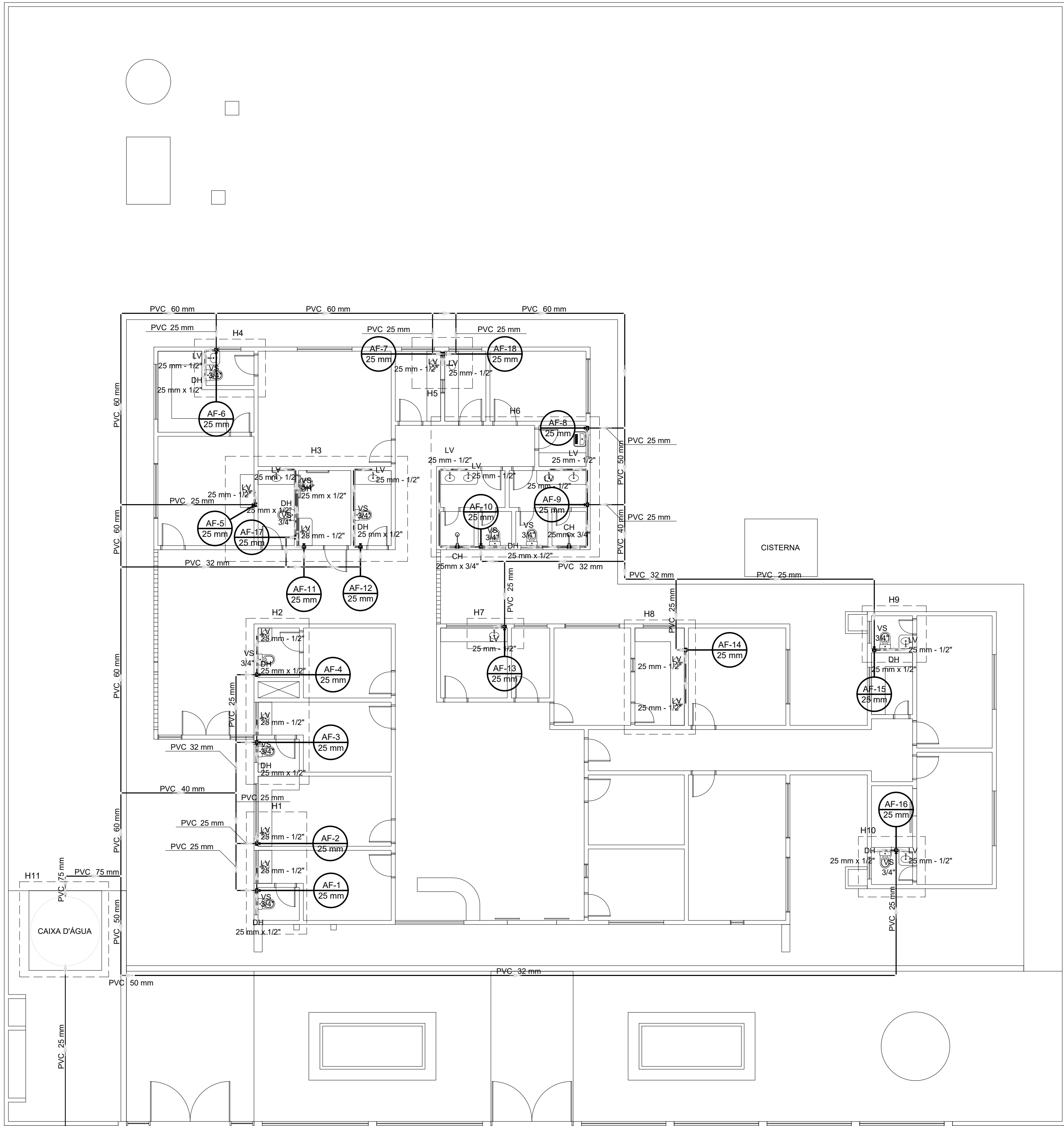
1 PLANTA TÉRREO Esc 1:100
