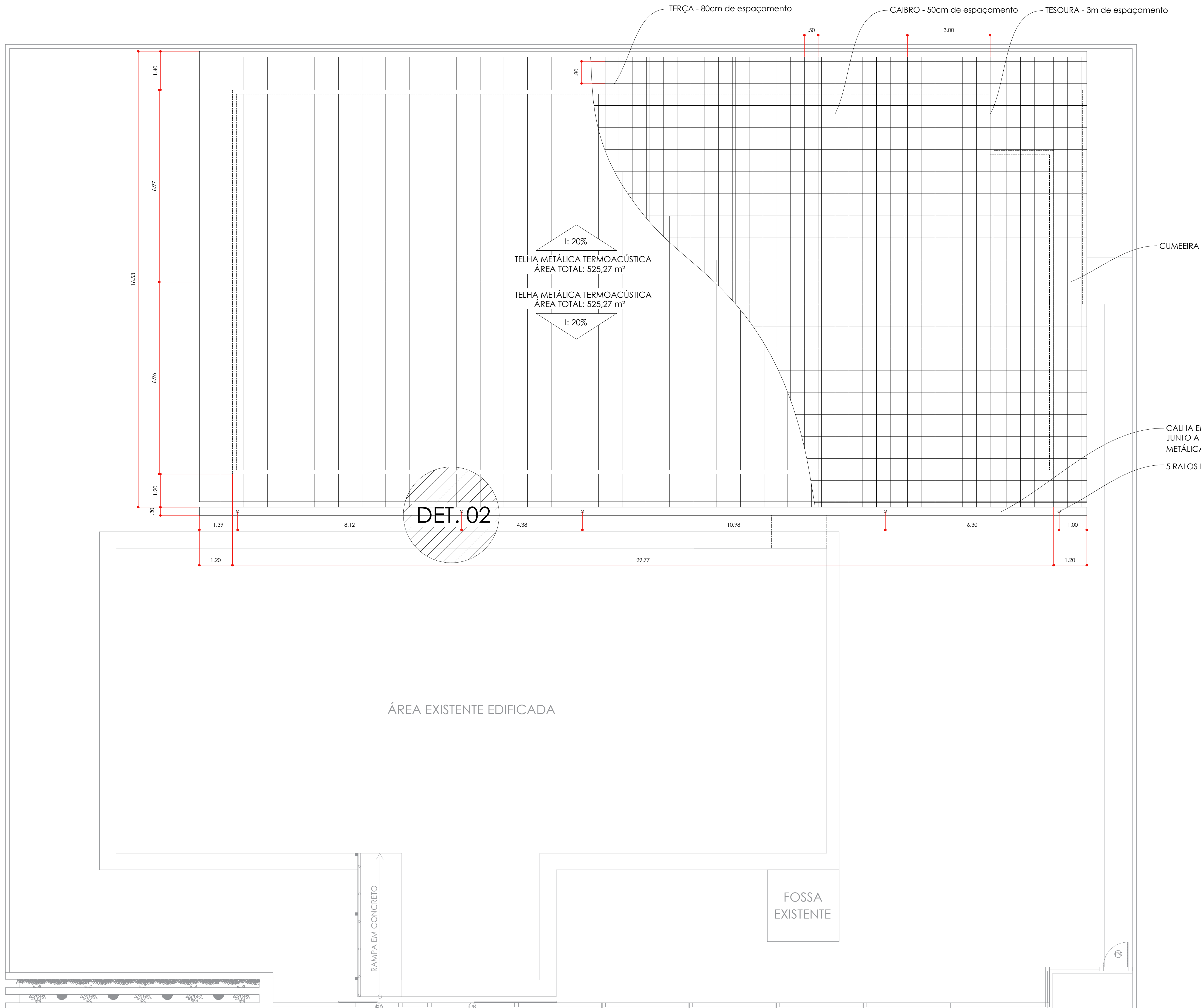
2 PLANTA DE COBERTURA - AMPLIAÇÃO ESCALA: 1:75
