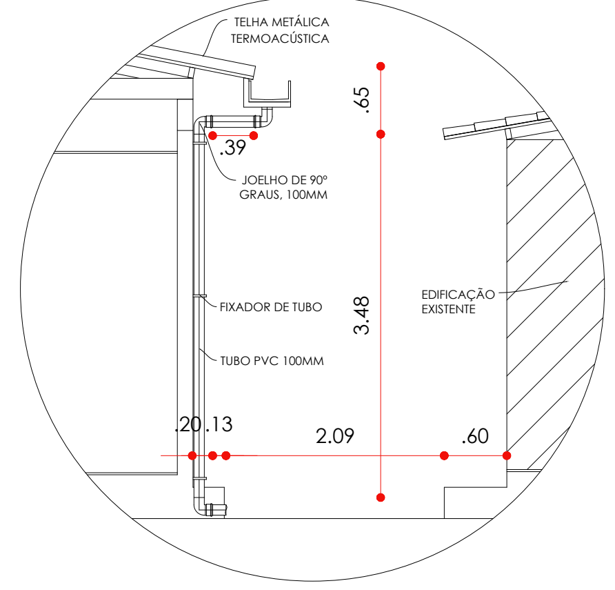
2 DETALHE 02 - DISTÂNCIA ENTRE OS BLOCOS S/ ESCALA
