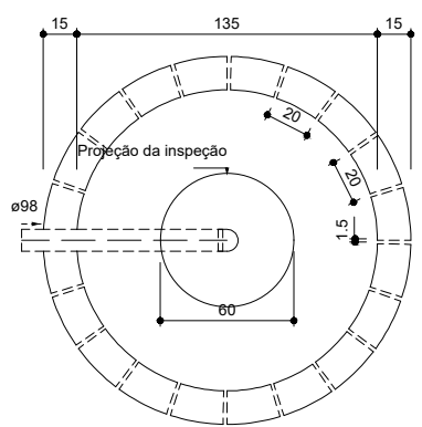
Sumidouro - Pavimento Planta baixa - ESC. 1:25
