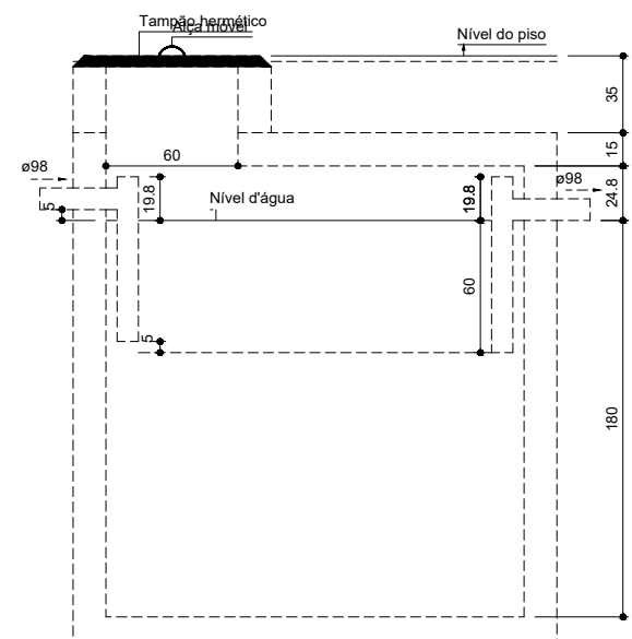
Tanque séptico - Pavimento Corte 1 - ESC. 1:25
