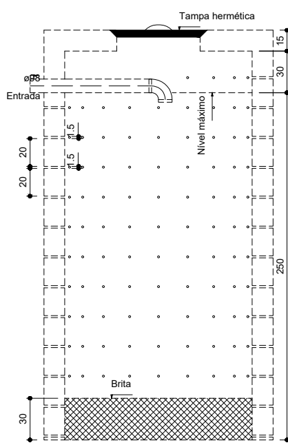
Sumidouro - Pavimento Corte 1 - ESC. 1:25
