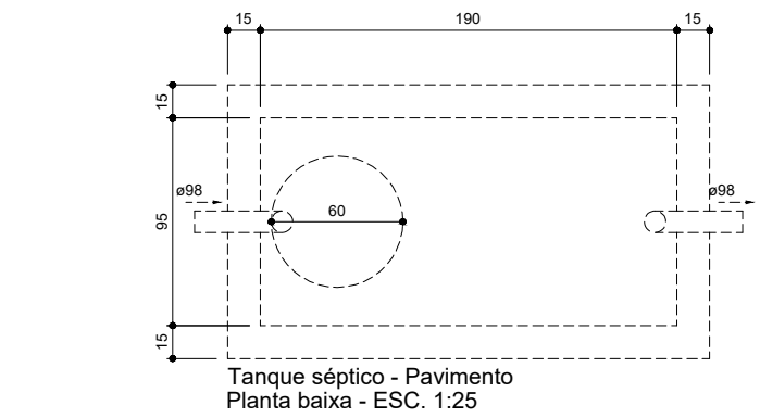
Tanque séptico - Pavimento Planta baixa - ESC. 1:25
