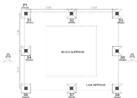
PLANTA DE PILARES
