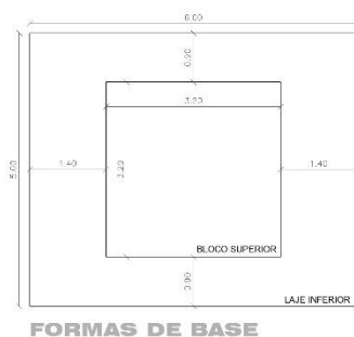
FORMAS DE BASE
