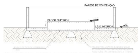
DETALHE DAS FERRAGENS
