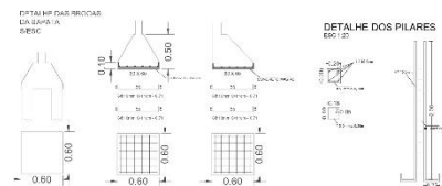
ARM. DE FERRAGENS DA BASE
