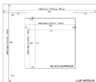
ARM. DE FERRAGENS DA BASE
